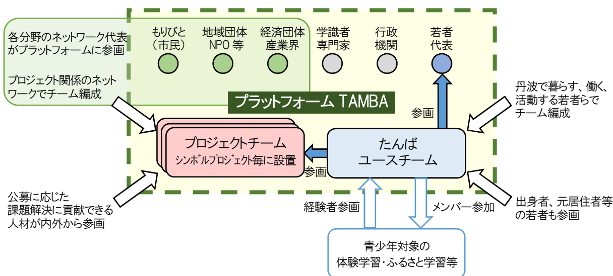
図8 推進体制のイメージ
