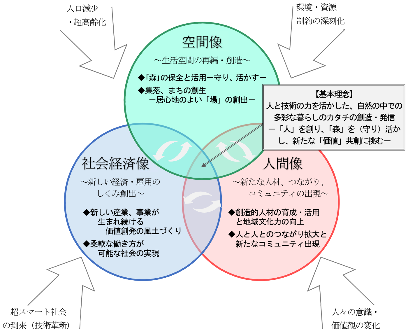
図7 「丹波 2050」の基本理念・地域社会像
