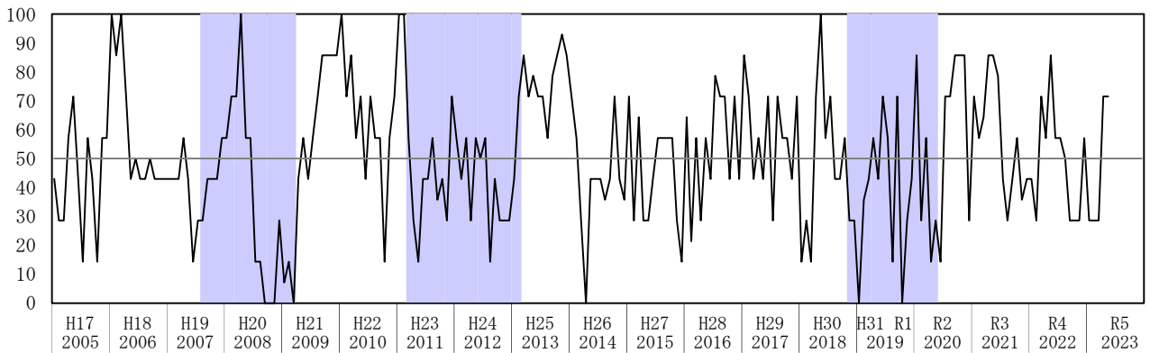
(1) 先行指数
