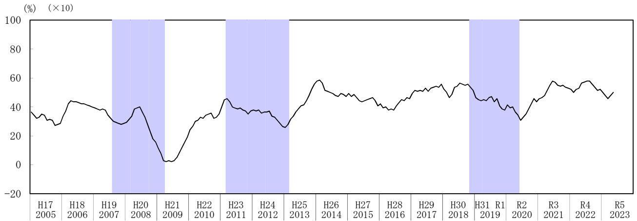
(1) 先行指数
