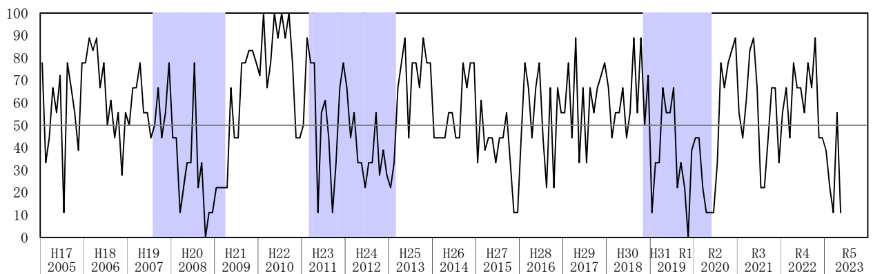
(2) 一致指数
