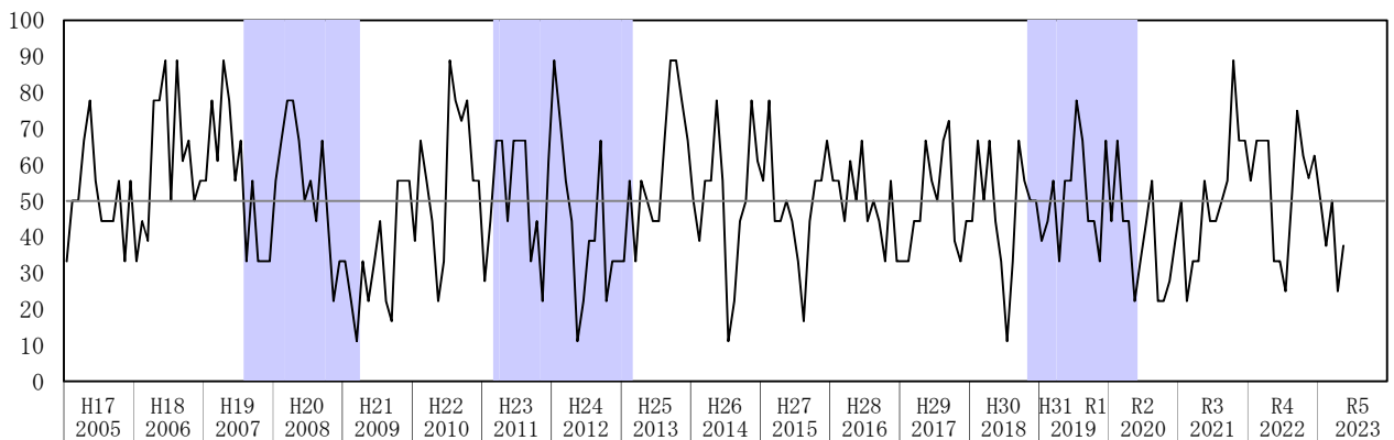
(3) 遅行指数
