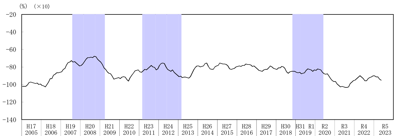
(3) 遅行指数
