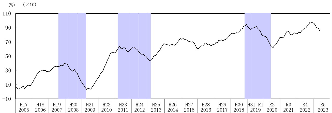
(2) 一致指数
