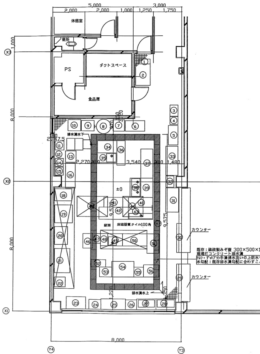
厨房平面詳細図 S=1/50
