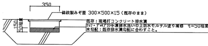
排水溝断面図 S=1/10
