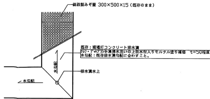
排水溝平面詳細図 S=1/10
