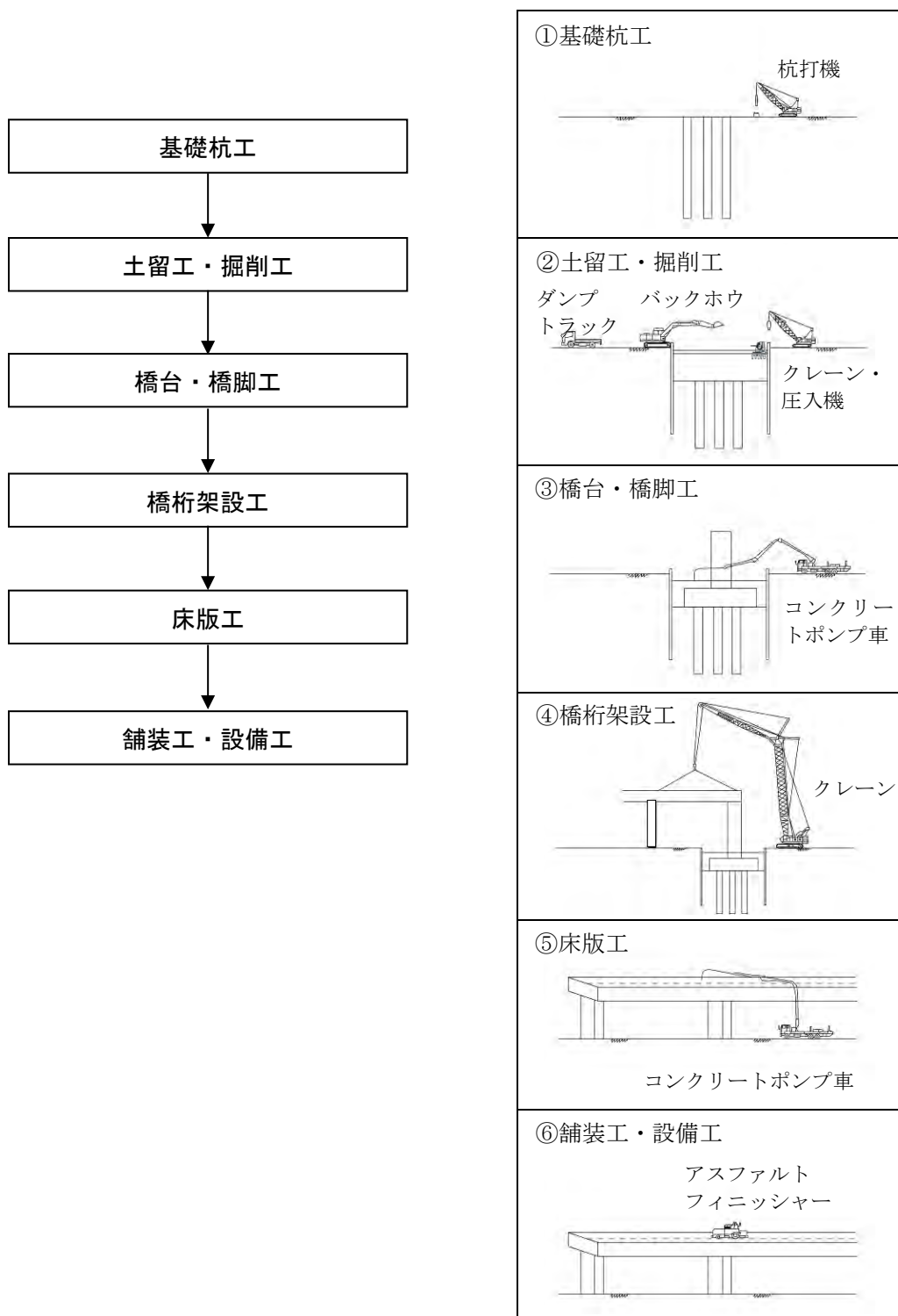
図 3-10 橋梁・高架工(陸上部)の施工順序
