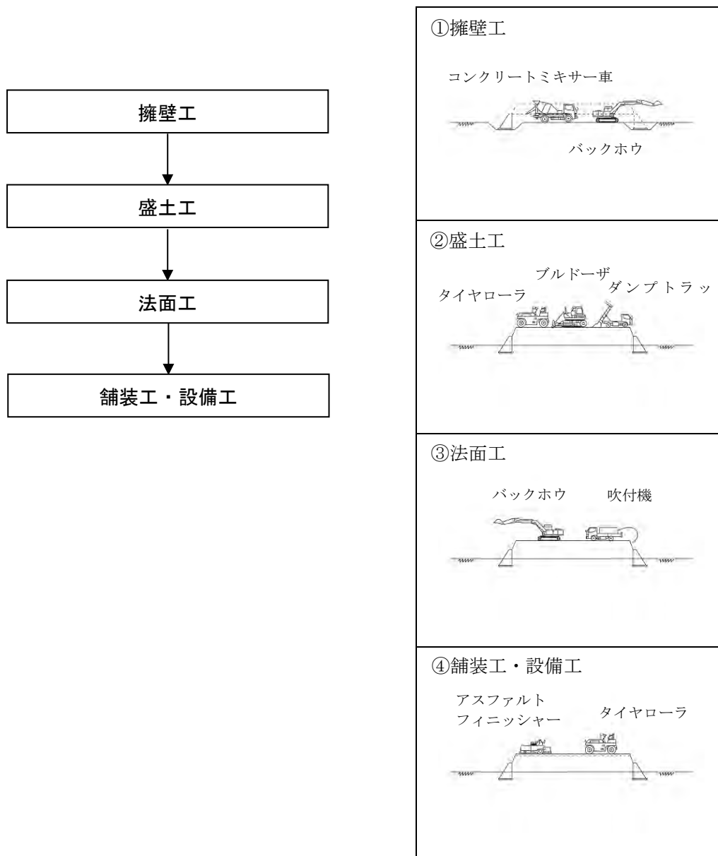
図 3-8 土工(盛土部)の施工順序
