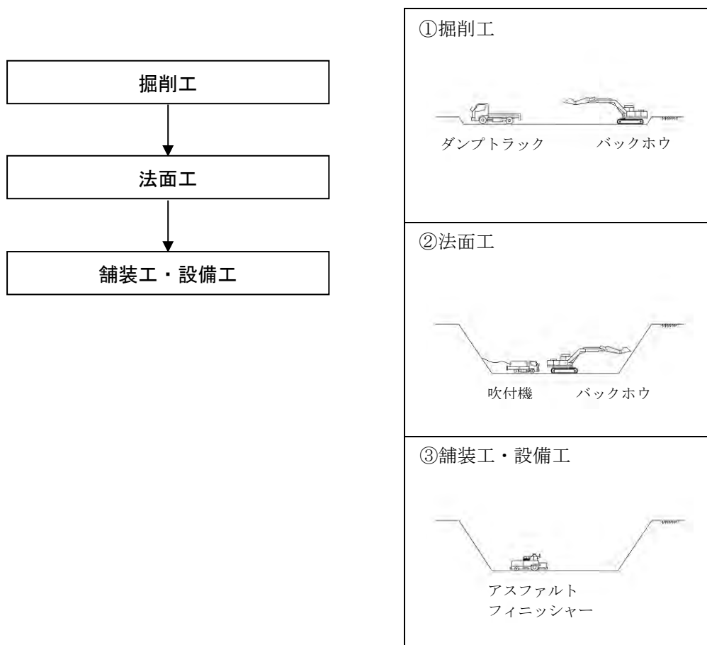
図 3-9 土工(切土部)の施工順序
