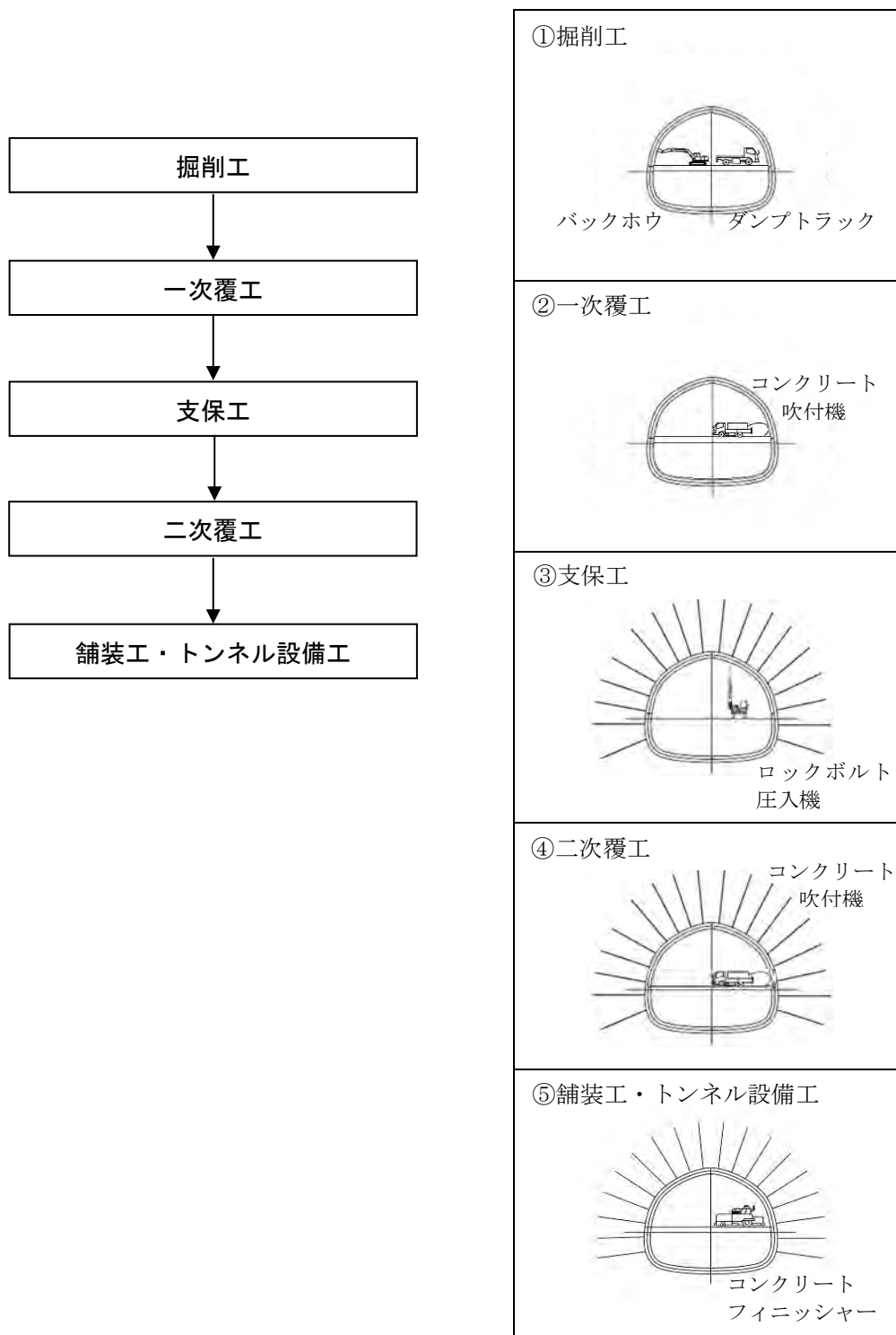
図 3-12 トンネル工の施工順序
