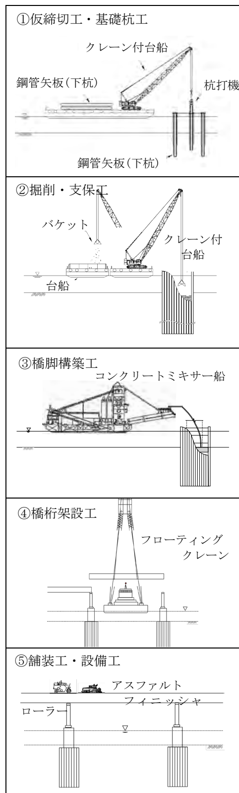
図 3-11 橋梁・高架工(河川内)の施工順序
