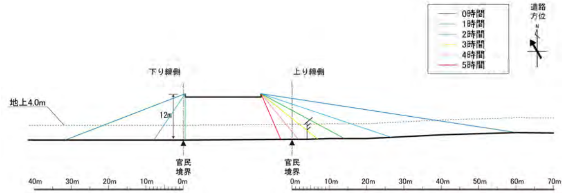
図 11.7-3(9) 日照障害の予測結果(予測地点 9 高砂市高砂町(1) 評価高さ：2階高さ(地上4.0m))
