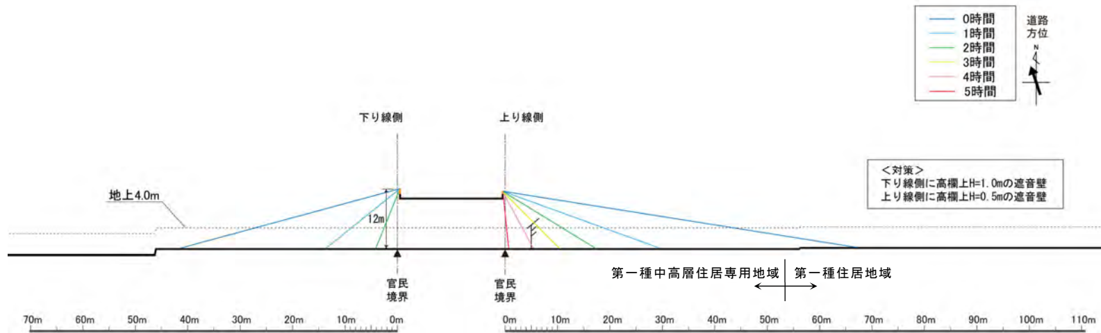
図 11.7-3(10) 日照障害の予測結果(予測地点 10 高砂市高砂町(2) 評価高さ：2階高さ(地上4.0m))
