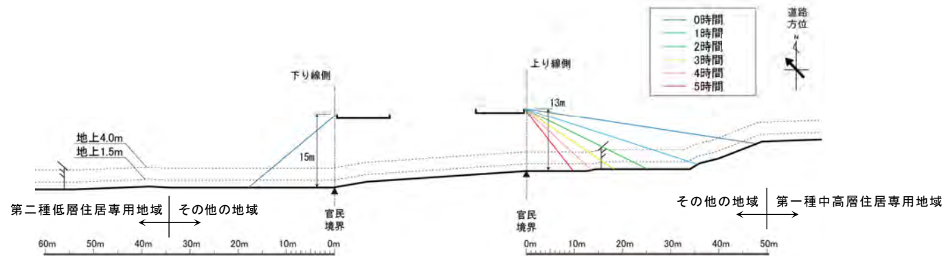
図 11.7-3(16) 日照障害の予測結果(予測地点 16 姫路市的形町の形(2) 評価高さ：2 階高さ(地上 4.0m)及び 1 階高さ(地上 1.5m))
