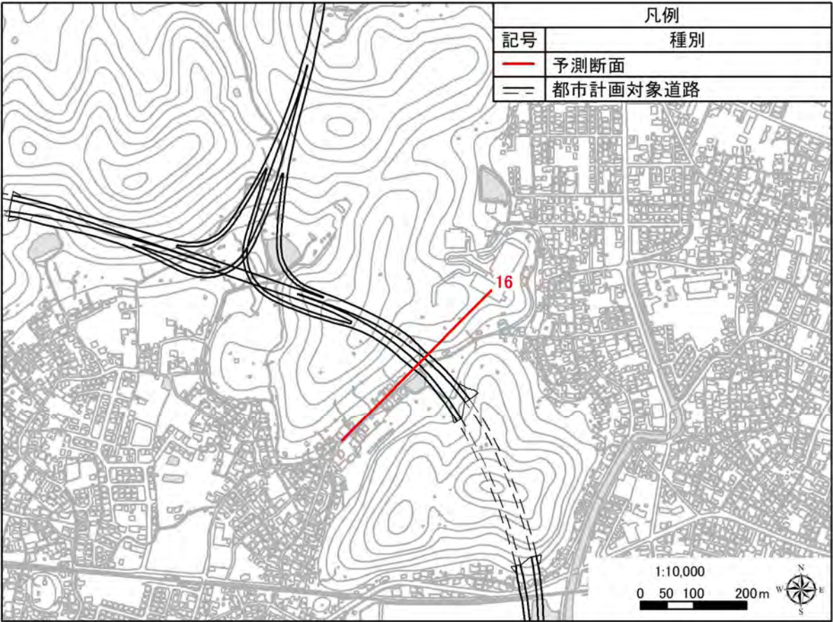
図 11.7-2(14) 日照阻害 予測地点図
