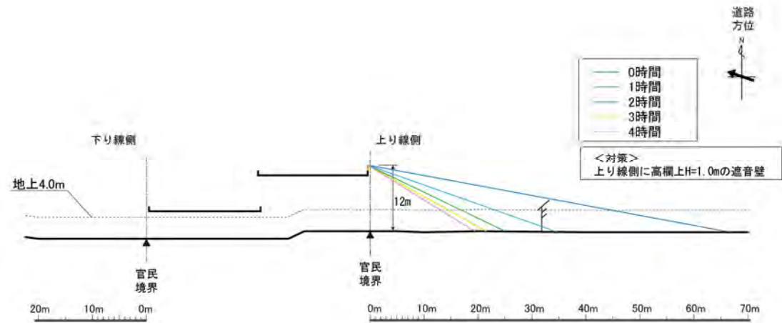
図 11.7-3(13) 日照障害の予測結果(予測地点 13 高砂市曾根町 評価高さ：2 階高さ(地上 4.0m))
