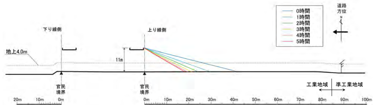
図 11. 7-3 (22) 日照障害の予測結果(予測地点 22 姫路市広畑区鶴町 評価高さ：2 階高さ(地上 4. 0m))
