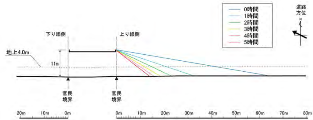
図 11.7-3(18) 日照障害の予測結果(予測地点 18 姫路市白浜町 評価高さ：2 階高さ(地上 4.0m))
