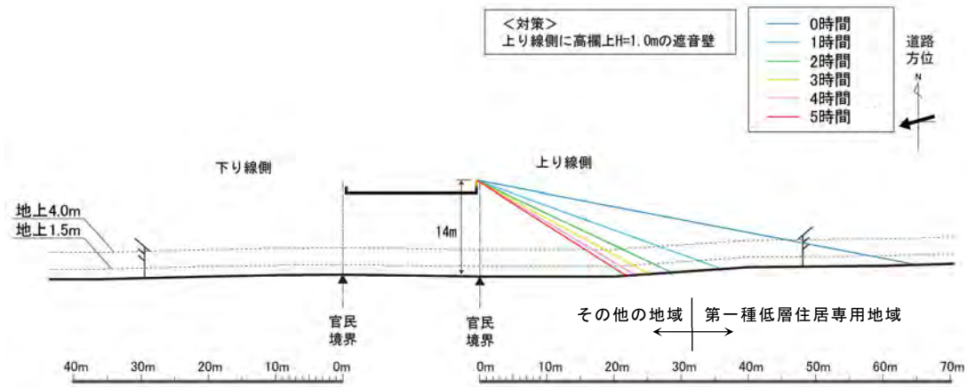
図 11.7-3(6) 日照障害の予測結果(予測地点 6 加古川市平岡町山之上 評価高さ：2 階高さ(地上 4.0m)及び 1 階高さ(地上 1.5m))
