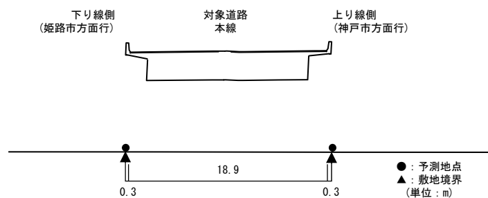
【予測断面図：予測地点 20】
