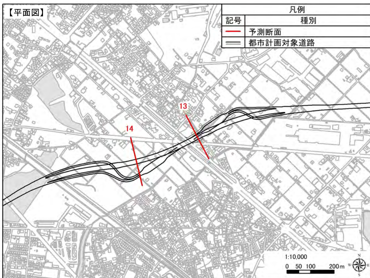
【予測断面図：予測地点 13】
