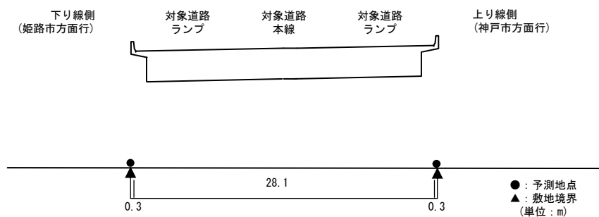
【予測断面図：予測地点 8】
