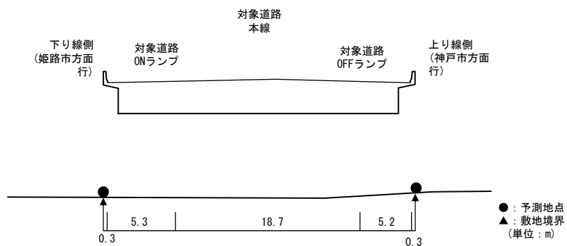
【予測断面図：予測地点 36】
