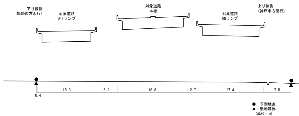
【予測断面図：予測地点 42】
