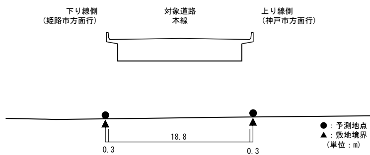
【予測断面図：予測地点 37】
