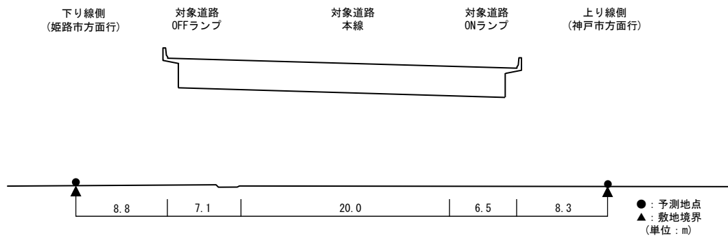
【予測断面図：予測地点 17】
