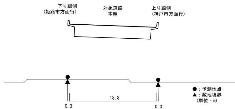
【予測断面図：予測地点 12】
