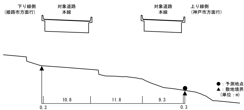
【予測断面図：予測地点 34】
