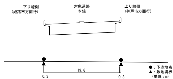
図 11.3-11 (23) 自動車の走行に係る振動 予測地点図
