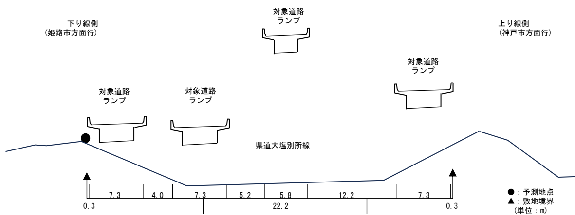
図 11.3-11(18) 自動車の走行に係る振動 予測地点図
