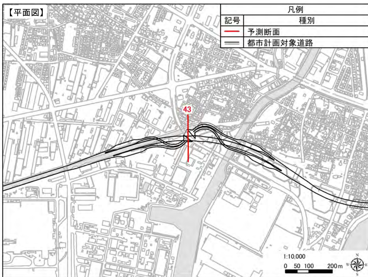
【予測断面図：予測地点 43】
