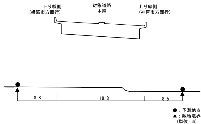
【予測断面図：予測地点 42】
