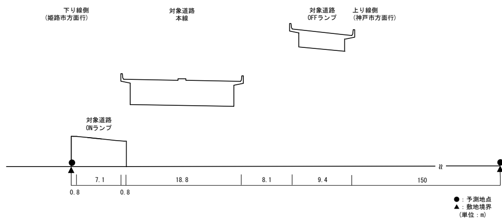
【予測断面図：予測地点 40】
