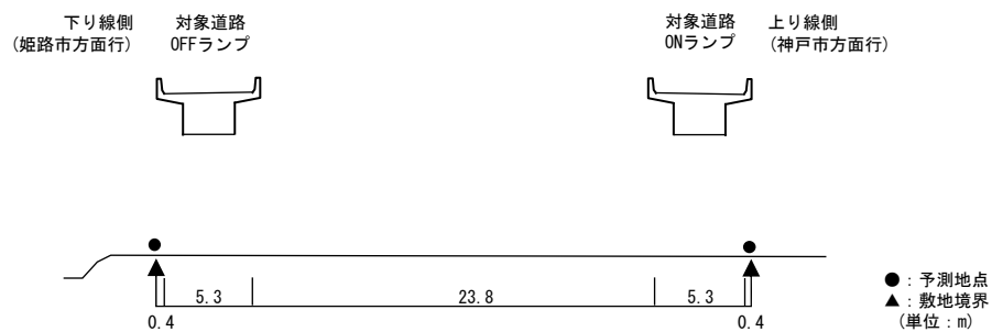
【予測断面図：予測地点 44】
