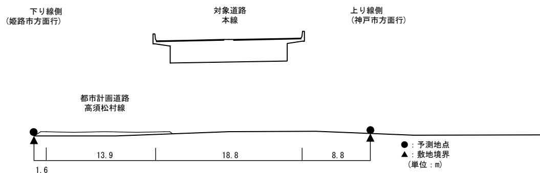
【予測断面図：予測地点 26】
