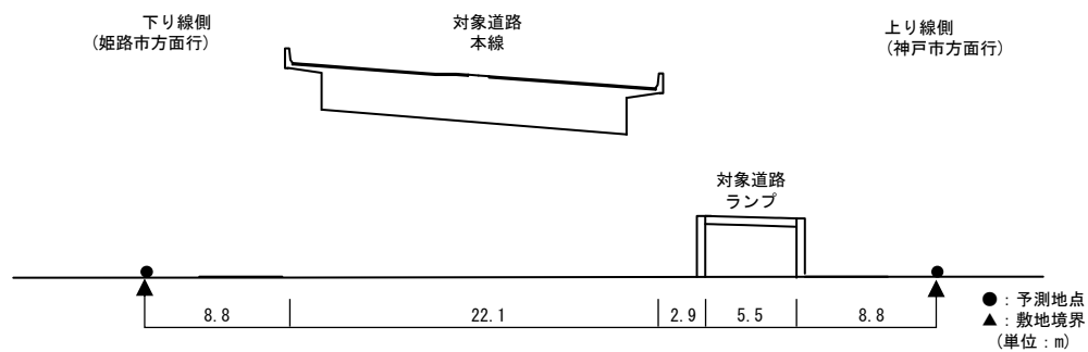
【予測断面図：予測地点 21】
