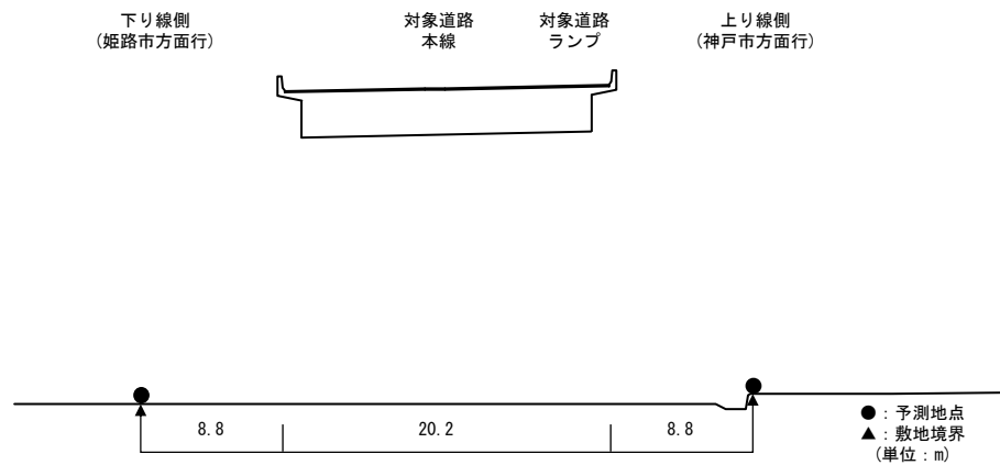
【予測断面図：予測地点 11】
