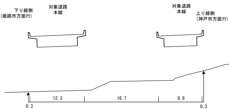
図 11.3-11(16) 自動車の走行に係る振動 予測地点図
