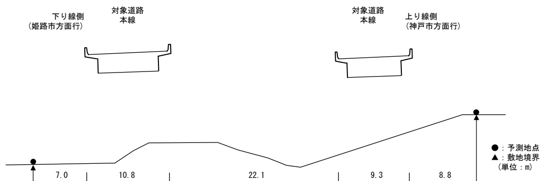
【予測断面図：予測地点 30】
