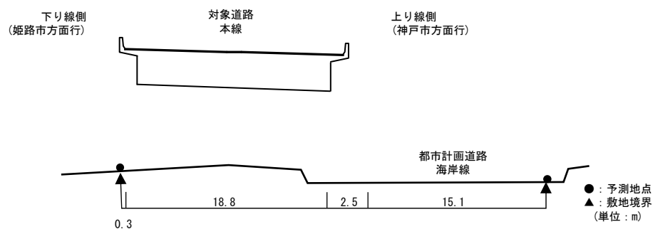
【予測断面図：予測地点 28】
