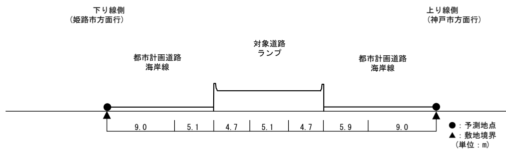
図 11.3-11 (20) 自動車の走行に係る振動 予測地点図
