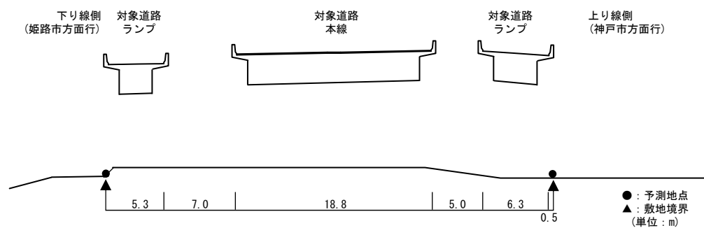
【予測断面図：予測地点 5】
