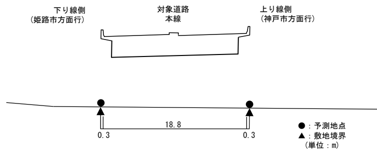
【予測断面図：予測地点 38】
