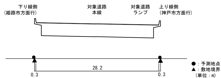
図 11.3-11(3) 自動車の走行に係る振動 予測地点図
