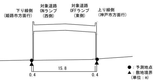
図 11.3-11(1) 自動車の走行に係る振動 予測地点図
