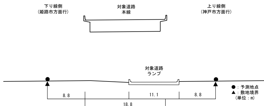
【予測断面図：予測地点 14】
