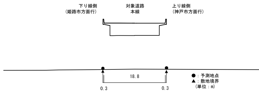
【予測断面図：予測地点 22】
