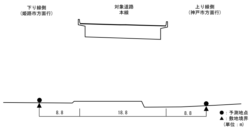
【予測断面図：予測地点 11】
