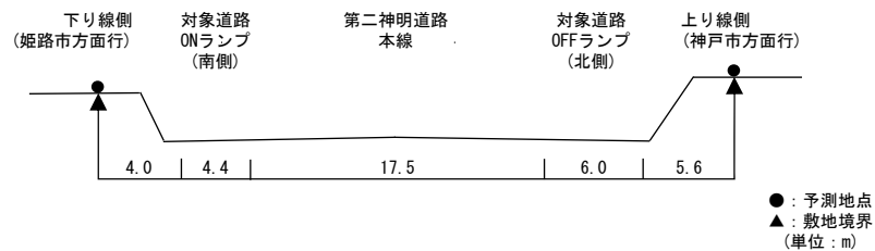
【予測断面図：予測地点 1】
