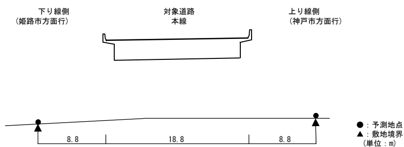
【予測断面図：予測地点 4】
