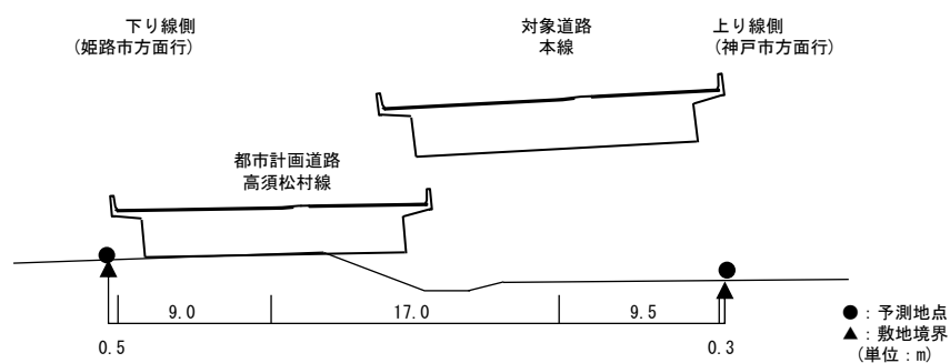
【予測断面図：予測地点 26】
