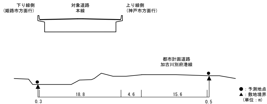
【予測断面図：予測地点 18】
