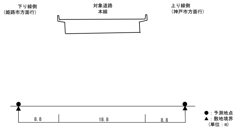
【予測断面図：予測地点 15】
