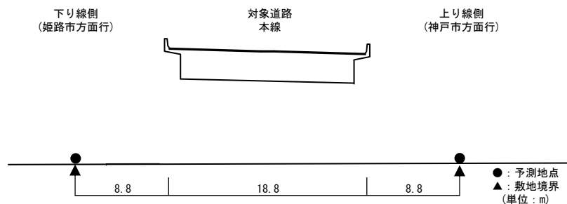
【予測断面図：予測地点 16】
