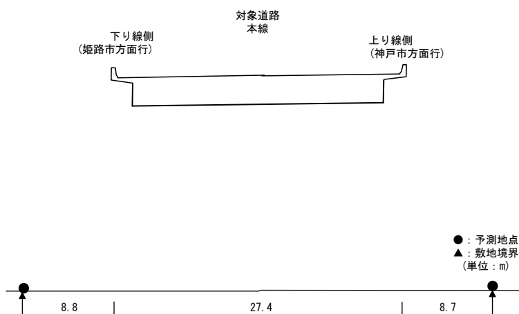
図 11.3-11(19) 自動車の走行に係る振動 予測地点図
