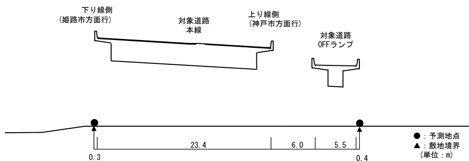
【予測断面図：予測地点 28】
