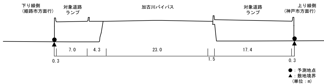
【予測断面図：予測地点 9】
