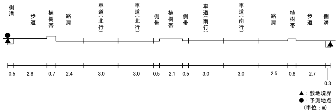
図 11.3-7(21) 予測断面(予測地点 21 姫路市広畑区正門通・市道幹第 43 号線)
