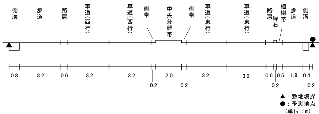
図 11.3-7(17) 予測断面(予測地点 17 姫路市飾磨区中島・一般国道 250 号)
