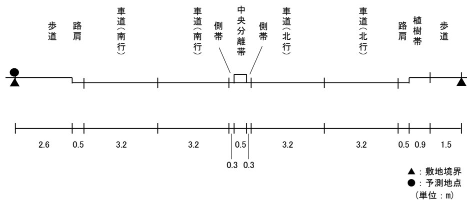
図 11.3-7(7) 予測断面(予測地点 7 加古川市金沢町・市道 48 号加古川別府港線)
