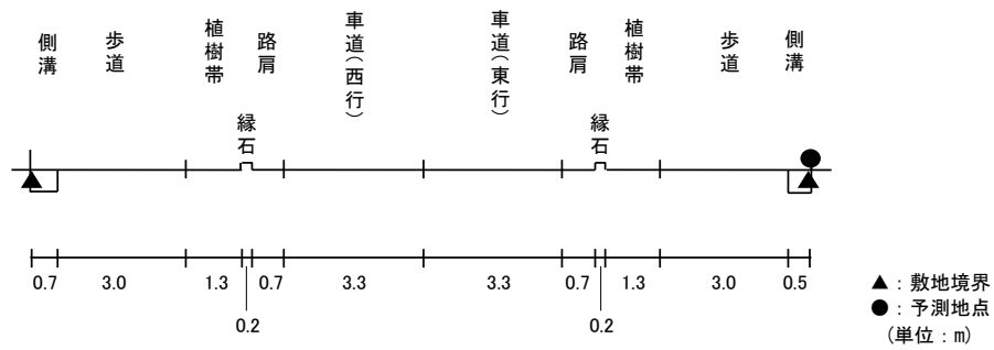
図 11.3-7(20) 予測断面(予測地点 20 姫路市広畑区長町・一般国道 250 号)
