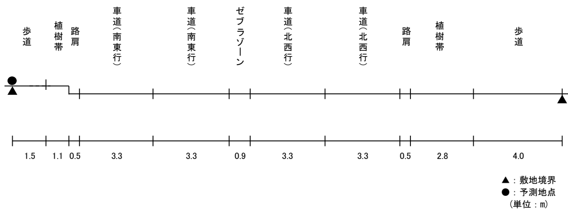
図 11.3-7(6) 予測断面(予測地点 6 加古川市別府町東町 ・市道 48 号加古川別府港線)
