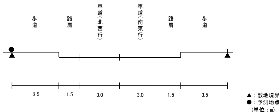
図 11.3-7(5) 予測断面(予測地点 5 播磨町宮西・町道 4 号浜幹線)
