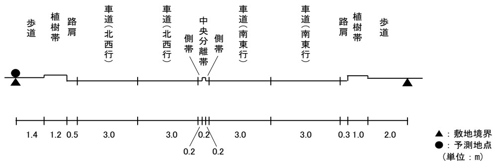
図 11.3-7(16) 予測断面(予測地点 16 姫路市白浜町(3)・市道白浜 149 号線)
