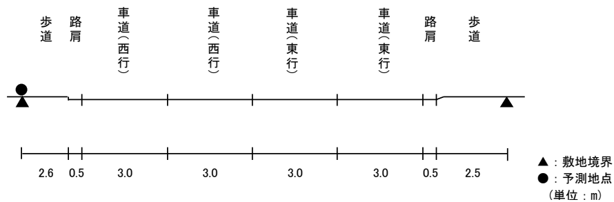
図 11.3-7(15) 予測断面(予測地点 15 姫路市白浜町(2)・一般国道 250 号)
