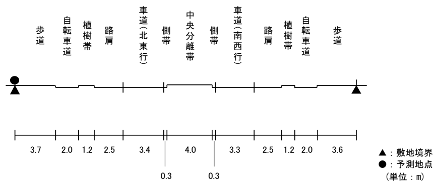
図 11.3-7(9) 予測断面(予測地点 9 高砂市梅井・一般県道 391 号伊保宝殿停車場線)
