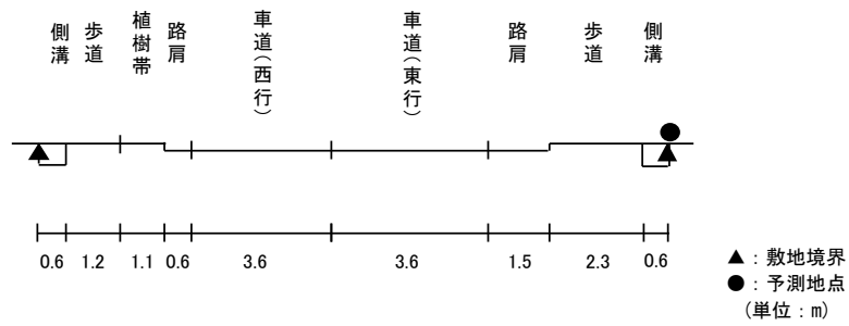
図 11.3-7(19) 予測断面(予測地点 19 姫路市飾磨区思案橋・一般国道 250 号)
