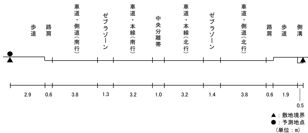
図 11.3-7(14) 予測断面(予測地点 14 姫路市白浜町(1)・一般国道 250 号)
