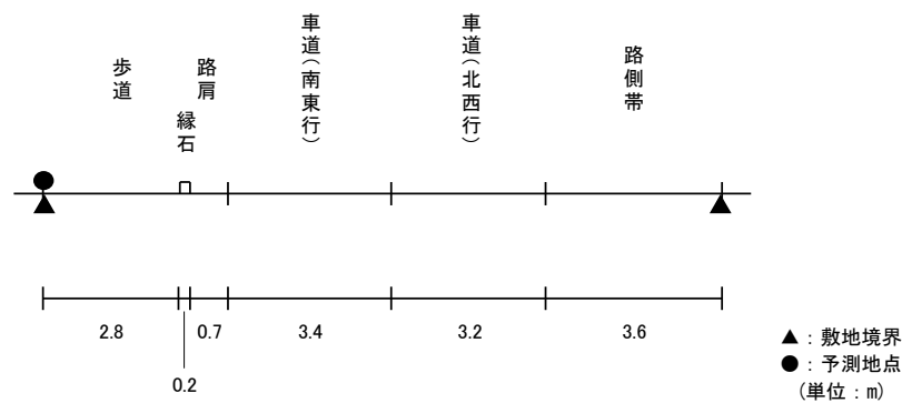
図 11.3-7(2) 予測断面(予測地点 2 加古川市平岡町高畑・一般国道 2 号)
