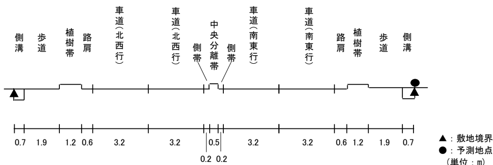
図 11.3-7(13) 予測断面(予測地点 13 姫路市木場前中町・市道幹第 55 号線)
