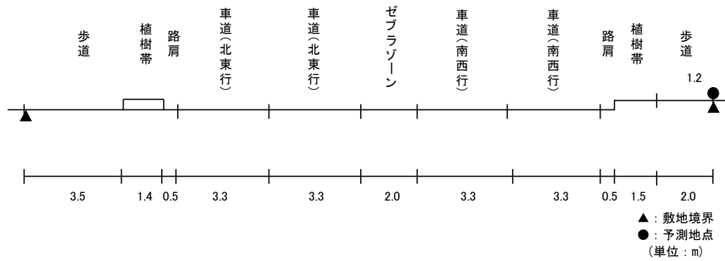
図 11.3-7(1) 予測断面(予測地点 1 稲美町六分一・主要地方道 84 号宗佐土山線)
