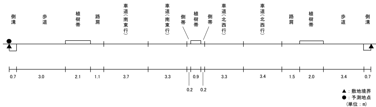
図 11.3-7(4) 予測断面(予測地点 4 加古川市平岡町中野・一般国道 250 号)
