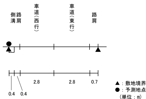
図 11.3-7(11) 予測断面(予測地点 11 姫路市の形町の形(1)・一般国道 250 号)
