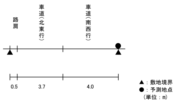
図 11.3-7(10) 予測断面(予測地点 10 高砂市曾根町・一般県道 555 号曾根阿弥陀線)
