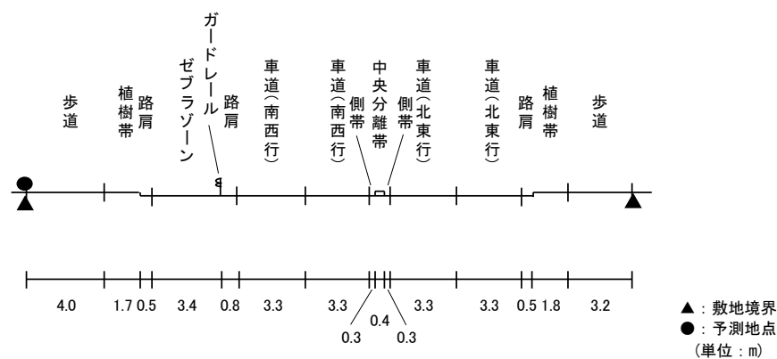
図 11.3-7(8) 予測断面(予測地点 8 高砂市荒井町東本町・主要地方道 43 号高砂北条線)
