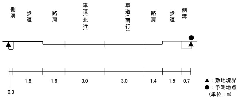
図 11.3-7(18) 予測断面(予測地点 18 姫路市飾磨区細江・一般国道 436 号)
