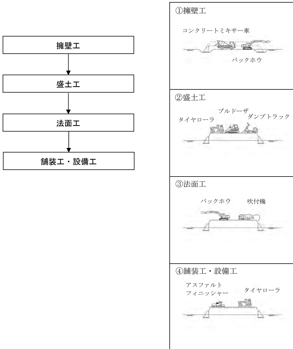
図 3.2-7 土工(盛土部)の施工順序
