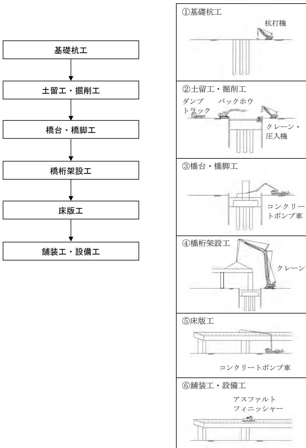
図 3.2-9 橋梁・高架工(陸上部)の施工順序
