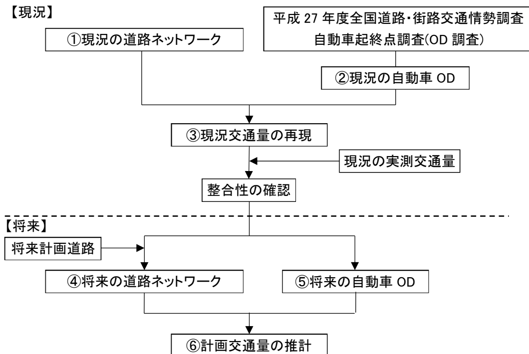
図 3.2-3 計画交通量の推計手順
