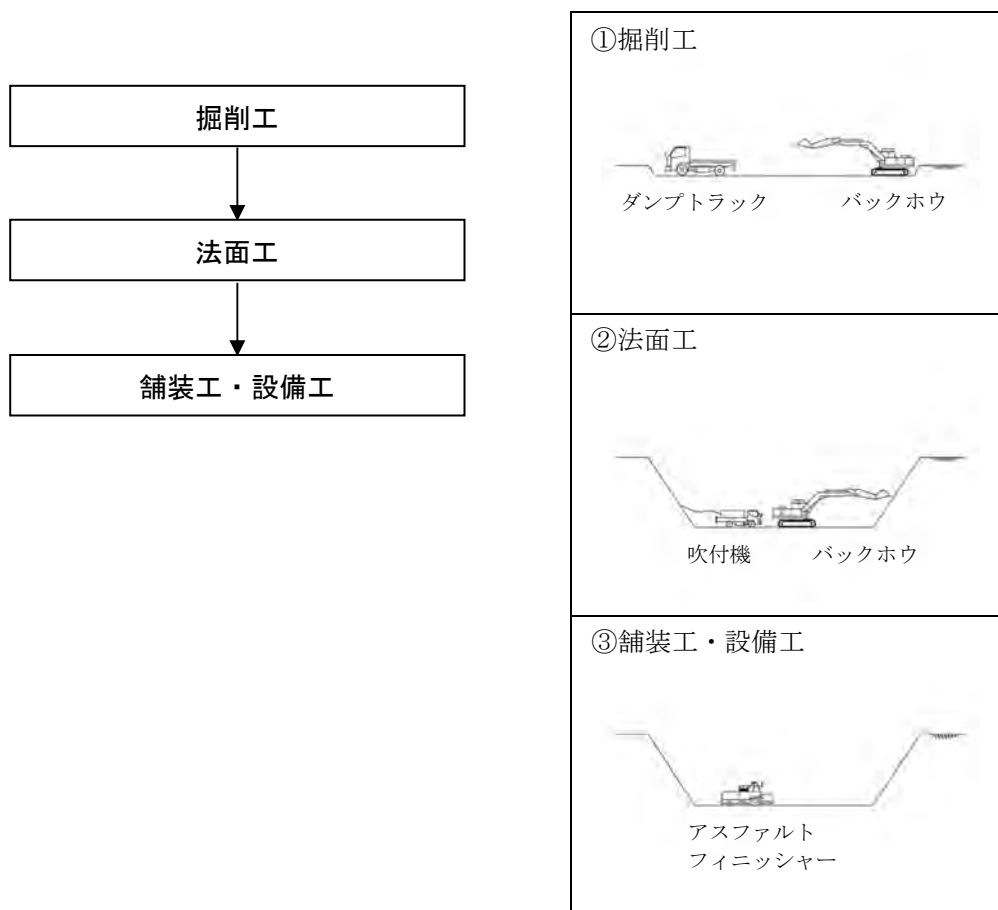
図 3.2-8 土工(切土部)の施工順序
