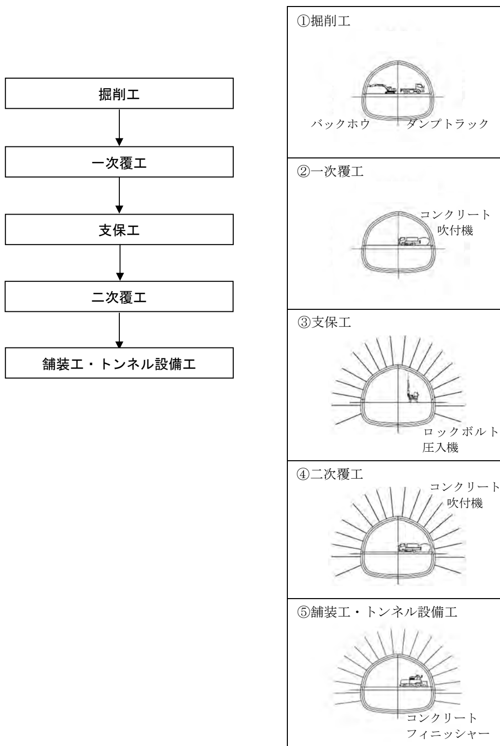
図 3.2-11 トンネル工の施工順序
