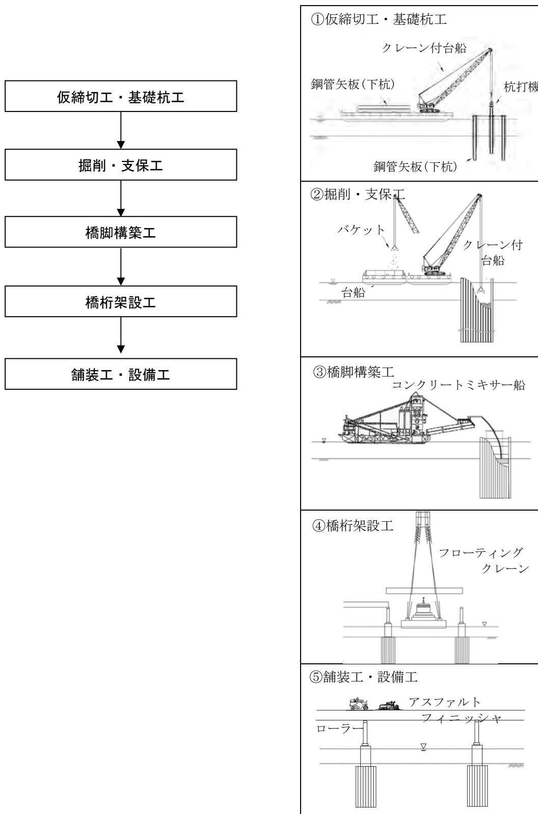
図 3.2-10 橋梁・高架工(河川内)の施工順序
