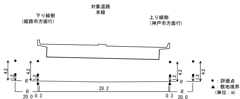
【予測断面図：断面 4-2】
