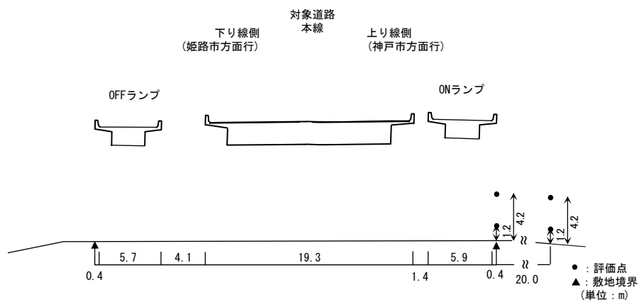
【予測断面図：断面 4-2】
