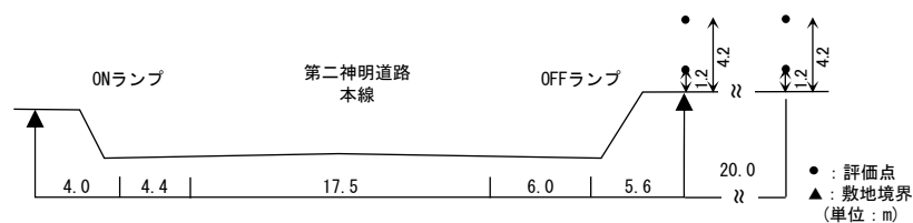
【予測断面図：断面 1-1】
