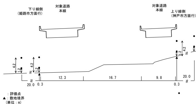
【予測断面図：断面 18-1】
