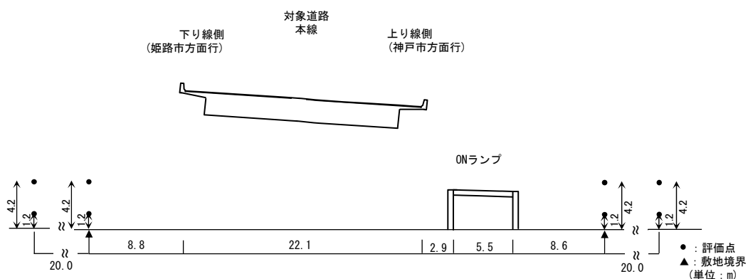
【予測断面図：断面 12-2】
