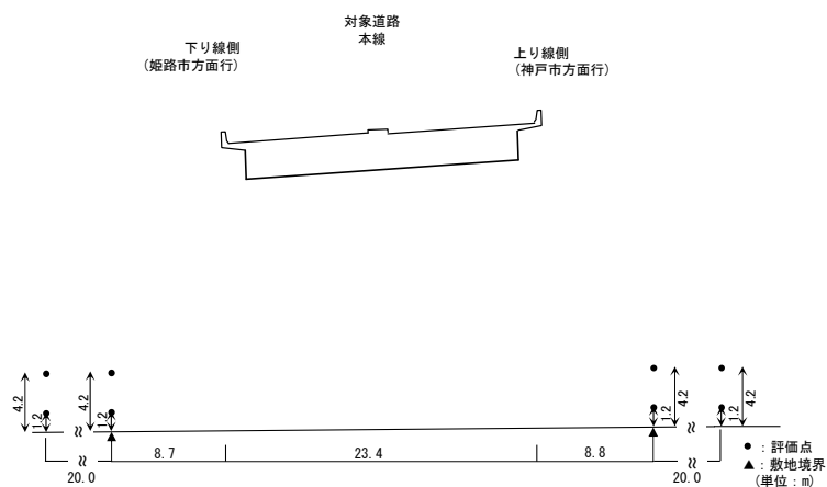
【予測断面図：断面 13-1】
