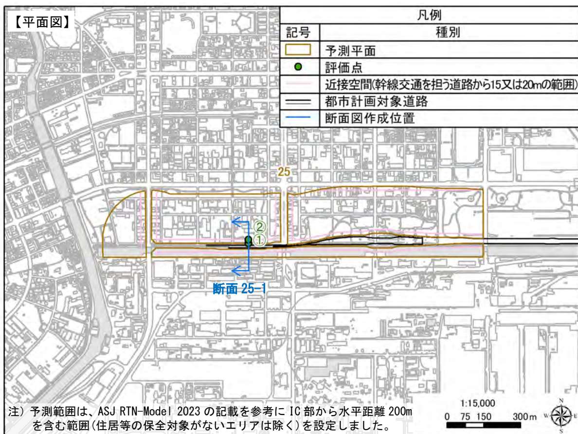
【予測断面図：断面 25-1】
