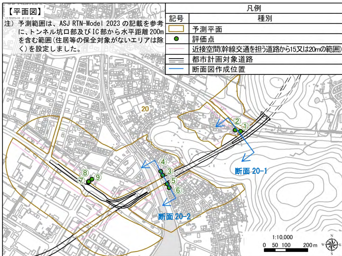
【予測断面図：断面 20-1】
