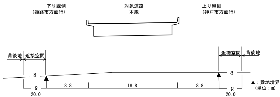
【予測断面図：予測地点 3】
