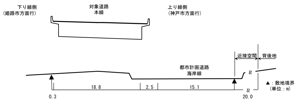
【予測断面図：予測地点 16】
