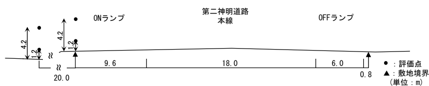
【予測断面図：断面 1-3】
