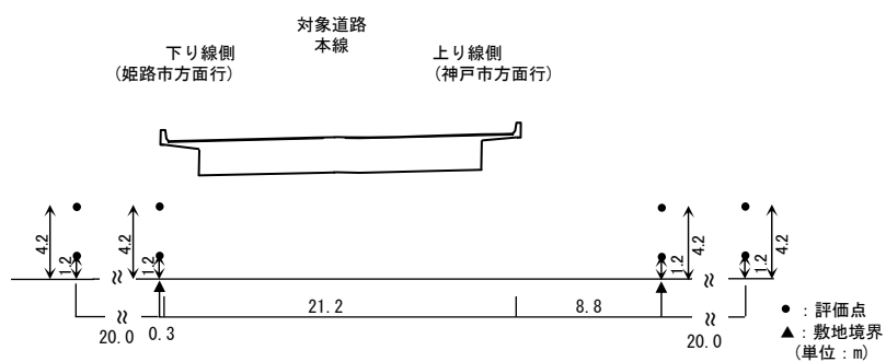
【予測断面図：断面 12-1】
