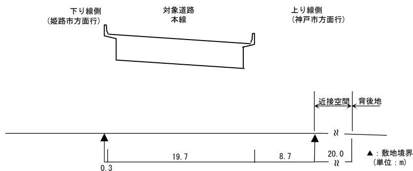
【予測断面図：予測地点 10】
