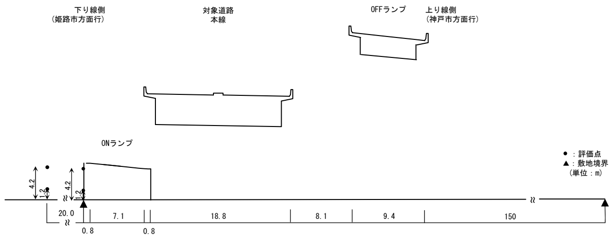
【予測断面図：断面 23-2】
