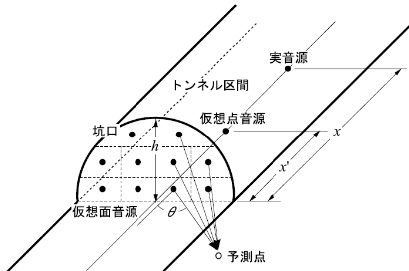
図 11.2-14 トンネル内の自動車と仮想音源の配置
