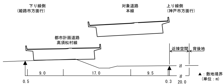
【予測断面図：予測地点 14】
