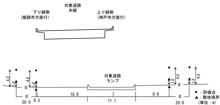
【予測断面図：断面 8-1】
