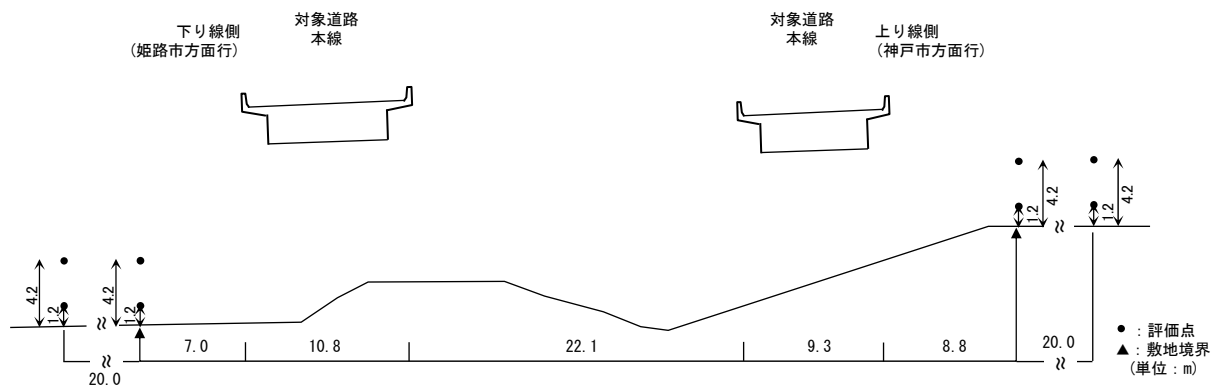
【予測断面図：断面 17-1】
