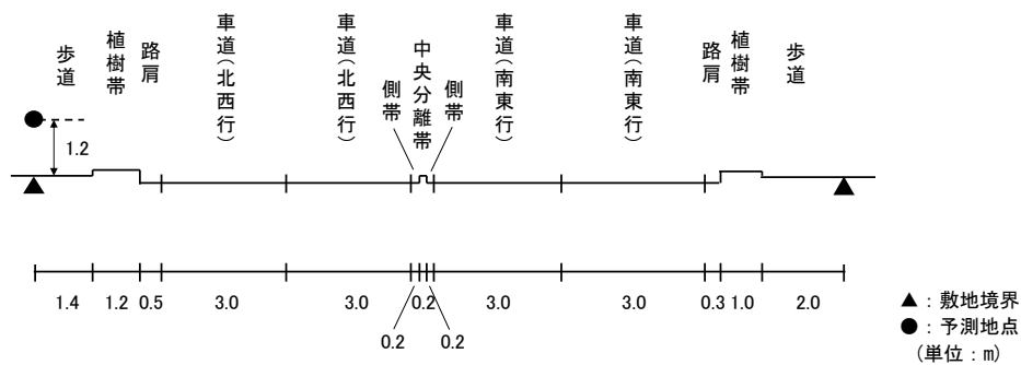
図 11.2-7(16) 予測断面(予測地点 16 姫路市白浜町(3)・市道白浜 149 号線)
