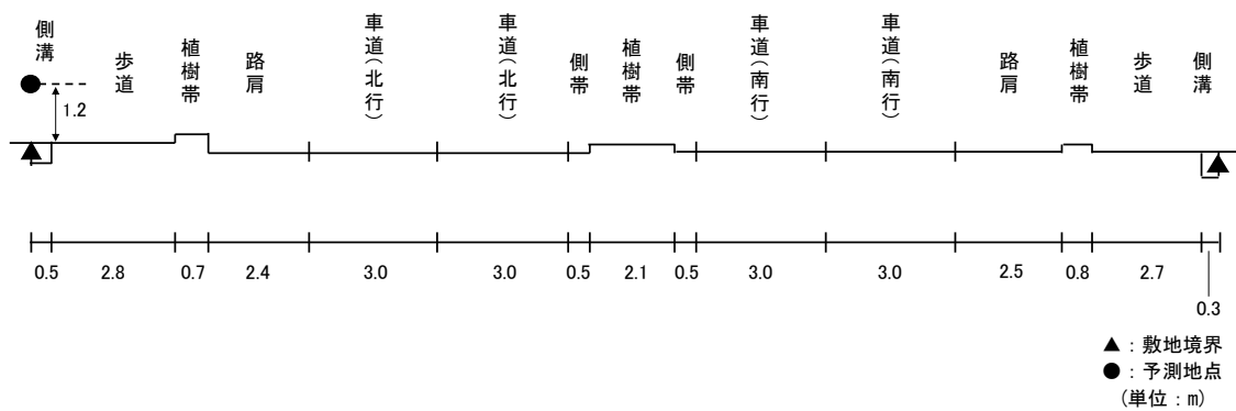
図 11.2-7(21) 予測断面(予測地点 21 姫路市広畑区正門通・市道幹第 43 号線)
