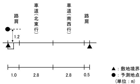
図 11.2-7(3) 予測断面(予測地点 3 加古川市平岡町・一般県道 382 号本荘平岡線)
