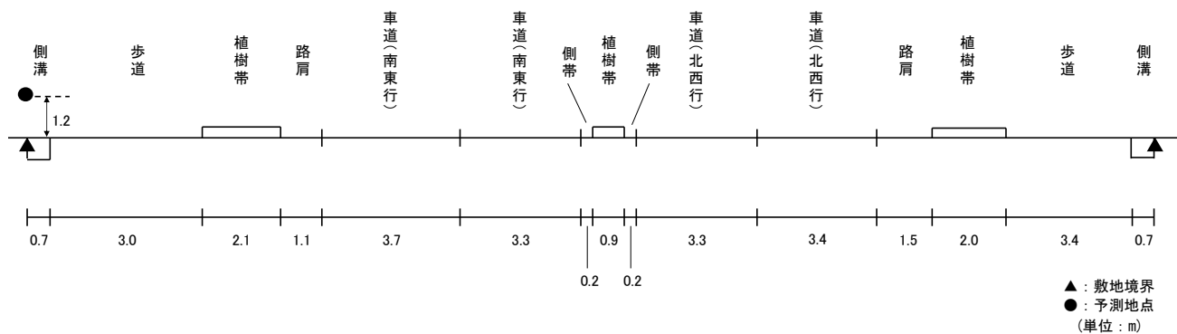
図 11.2-7(4) 予測断面(予測地点 4 加古川市平岡町中野・一般国道 250 号)
