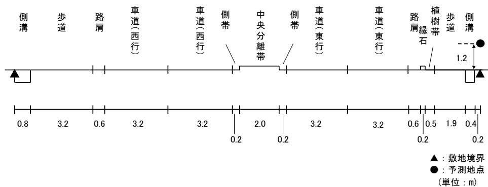
図 11.2-7(17) 予測断面(予測地点 17 姫路市飾磨区中島・一般国道 250 号)
