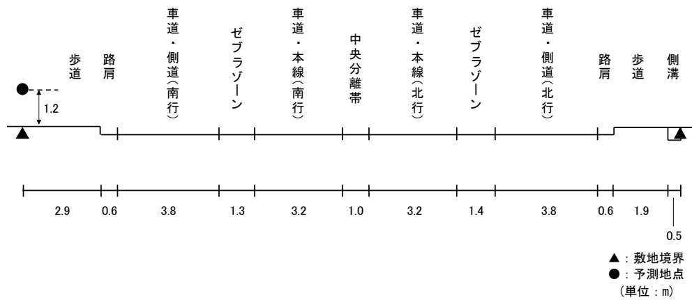
図 11.2-7(14) 予測断面(予測地点 14 姫路市白浜町(1)・一般国道 250 号)
