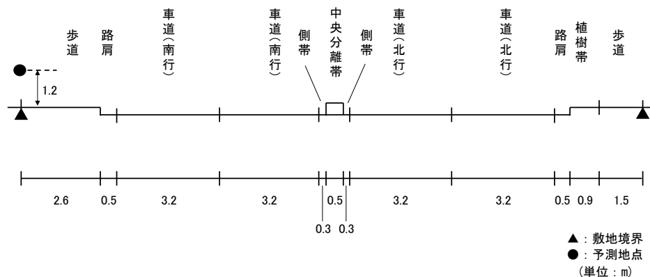
図 11.2-7(7) 予測断面(予測地点 7 加古川市金沢町・市道 48 号加古川別府港線)
