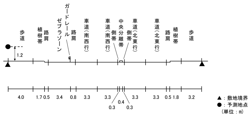
図 11.2-7(8) 予測断面(予測地点 8 高砂市荒井町東本町・主要地方道 43 号高砂北条線)
