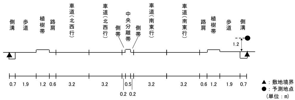
図 11.2-7(13) 予測断面(予測地点 13 姫路市木場前中町・市道幹第 55 号線)
