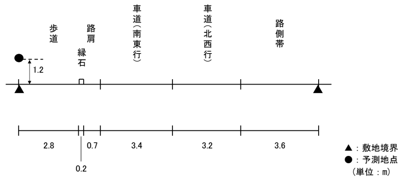
図 11.2-7(2) 予測断面(予測地点 2 加古川市平岡町高畑・一般国道 2 号)
