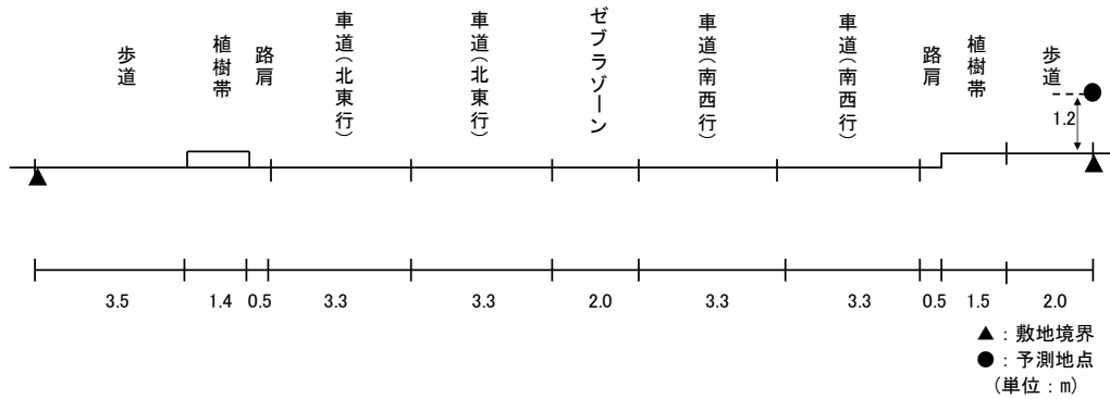
図 11.2-7(1) 予測断面(予測地点 1 稲美町六分一・主要地方道 84 号宗佐土山線)
