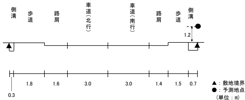
図 11.2-7(18) 予測断面(予測地点 18 姫路市飾磨区細江・一般国道 436 号)
