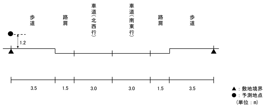
図 11.2-7(5) 予測断面(予測地点 5 播磨町宮西・町道 4 号浜幹線)
