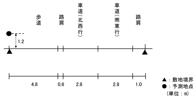
図 11.2-7(12) 予測断面(予測地点 12 姫路市の形町の形(2)・一般県道 399 号大塩別所線)
