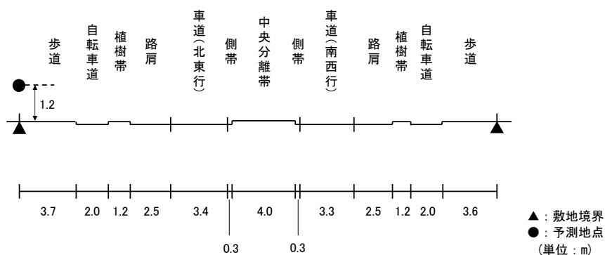
図 11.2-7(9) 予測断面(予測地点 9 高砂市梅井・一般県道 391 号伊保宝殿停車場線)
