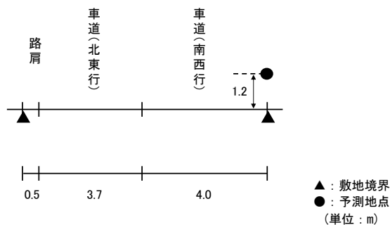
図 11.2-7(10) 予測断面(予測地点 10 高砂市曾根町・一般県道 555 号曾根阿弥陀線)
