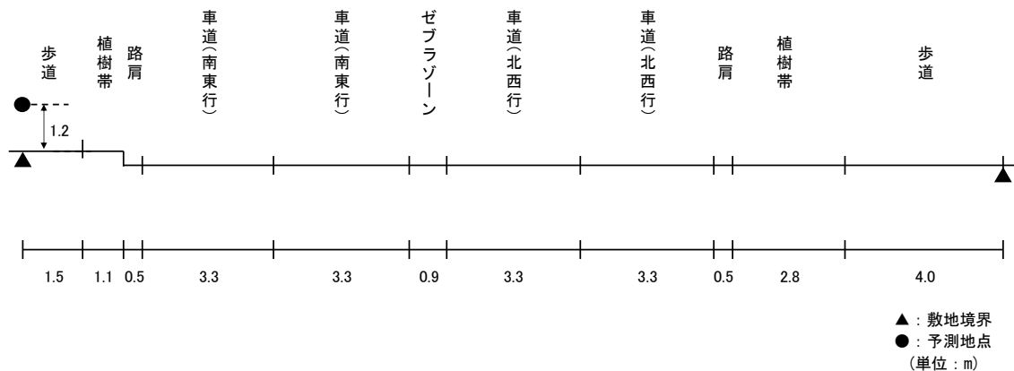
図 11.2-7(6) 予測断面(予測地点 6 加古川市別府町東町・市道 48 号加古川別府港線)
