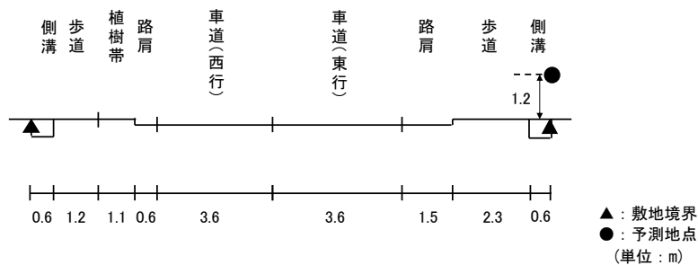
図 11.2-7(19) 予測断面(予測地点 19 姫路市飾磨区思案橋・一般国道 250 号)
