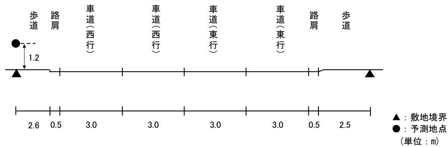
図 11.2-7(15) 予測断面(予測地点 15 姫路市白浜町(2)・一般国道 250 号)
