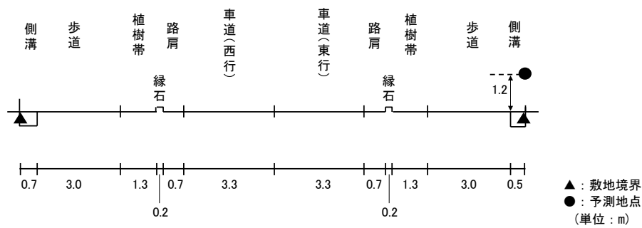
図 11.2-7(20) 予測断面(予測地点 20 姫路市広畑区長町・一般国道 250 号)
