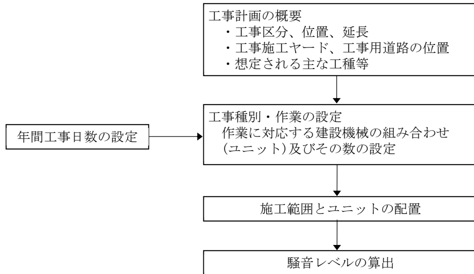
図 11. 2-2 建設機械の稼働に係る騒音の予測手順
