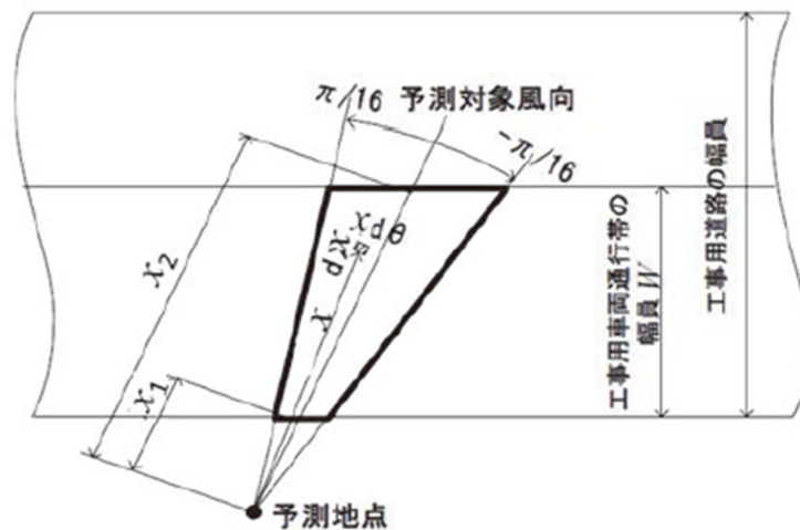
図 11.1-23 風向別の発生源の範囲と予測地点の距離の考え方
