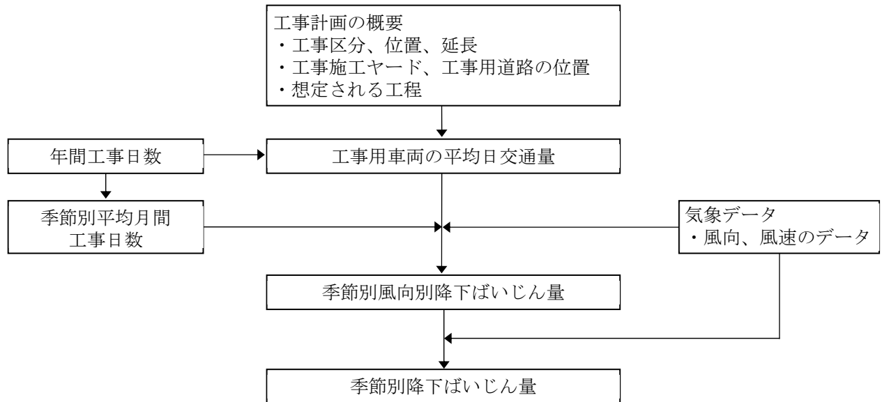
図 11. 1-22 工事用車両の運行に係る粉じん等の予測手順
