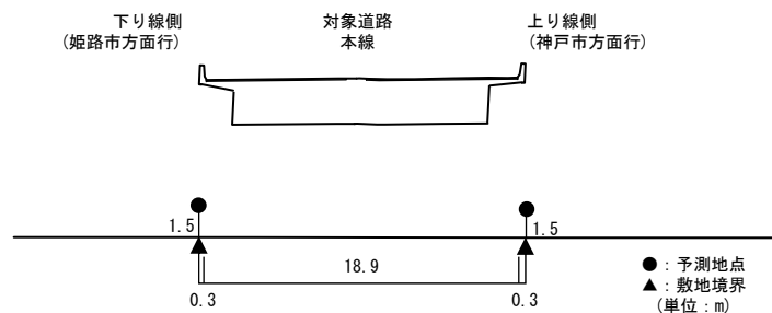
図 11.1-16(9) 自動車の走行に係る二酸化窒素及び浮遊粒子状物質 予測地点図
