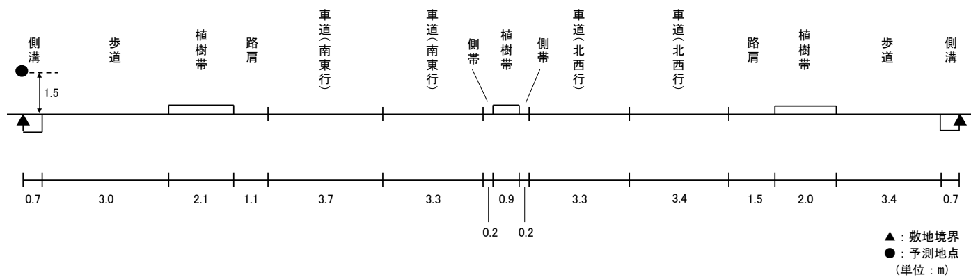
図 11.1-9(4) 予測断面図(予測地点 4 加古川市平岡町中野・一般国道 250 号)
