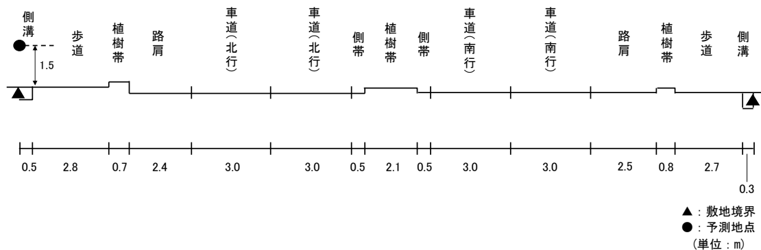
図 11.1-9(21) 予測断面図(予測地点 21 姫路市広畑区正門通・市道幹第 43 号線)
