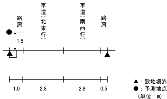
図 11.1-9(3) 予測断面図(予測地点 3 加古川市平岡町・一般県道 382 号本荘平岡線)
