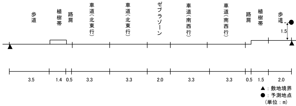
図 11.1-9(1) 予測断面図(予測地点 1 稲美町六分一・主要地方道 84 号宗佐土山線)
