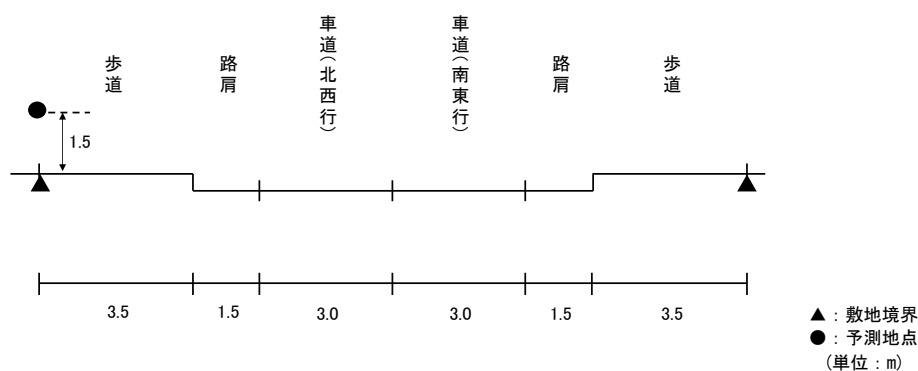
図 11.1-9(5) 予測断面図(予測地点 5 播磨町宮西・町道 4 号浜幹線)
