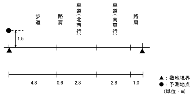
図 11.1-9(12) 予測断面図(予測地点 12 姫路市の形町の形(2)・一般県道 399 号大塩別所線)
