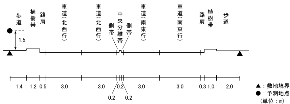
図 11.1-9(16) 予測断面図(予測地点 16 姫路市白浜町(3)・市道白浜 149 号線)
