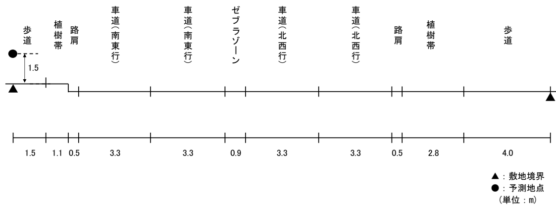
図 11.1-9(6) 予測断面図(予測地点 6 加古川市別府町東町 ・市道 48 号加古川別府港線)
