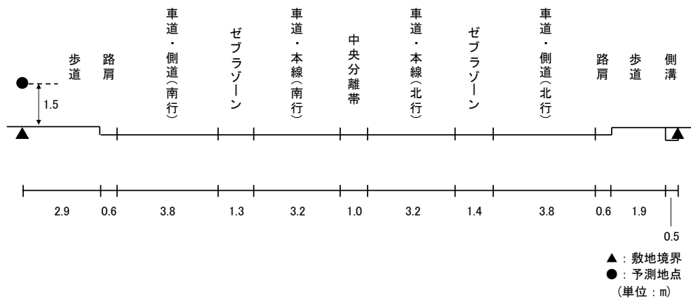
図 11.1-9(14) 予測断面図(予測地点 14 姫路市白浜町(1)・一般国道 250 号)
