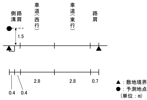
図 11.1-9(11) 予測断面図(予測地点 11 姫路市の形町の形(1)・一般国道 250 号)
