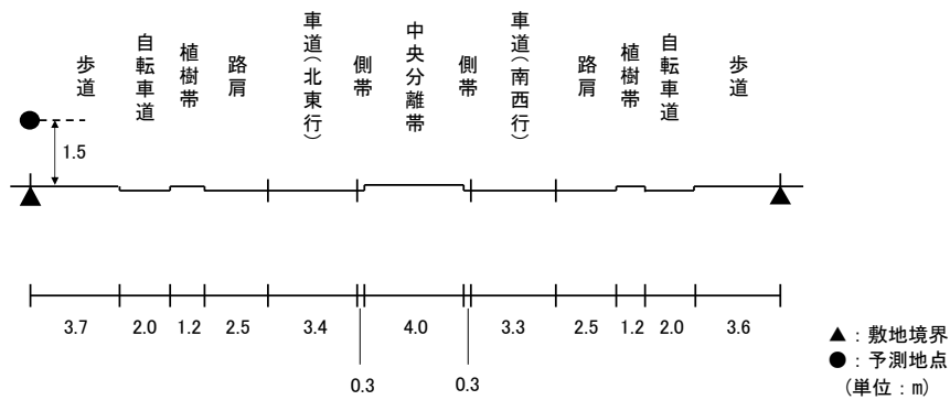
図 11.1-9(9) 予測断面図(予測地点 9 高砂市梅井・一般県道 391 号伊保宝殿停車場線)
