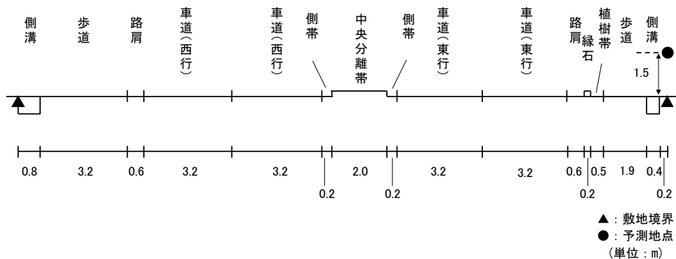
図 11.1-9(17) 予測断面図(予測地点 17 姫路市飾磨区中島・一般国道 250 号)
