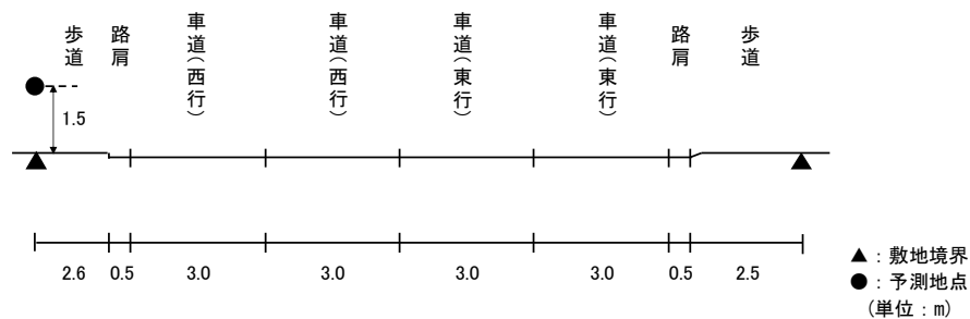
図 11.1-9(15) 予測断面図(予測地点 15 姫路市白浜町(2)・一般国道 250 号)
