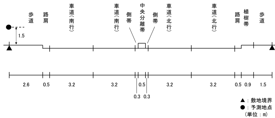
図 11.1-9(7) 予測断面図(予測地点 7 加古川市金沢町・市道 48 号加古川別府港線)
