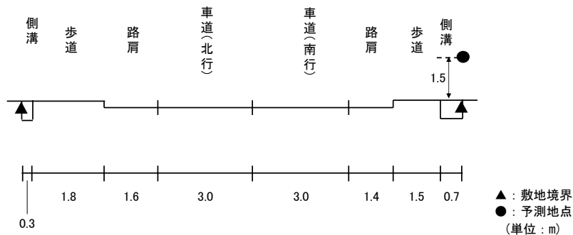
図 11.1-9(18) 予測断面図(予測地点 18 姫路市飾磨区細江・一般国道 436 号)
