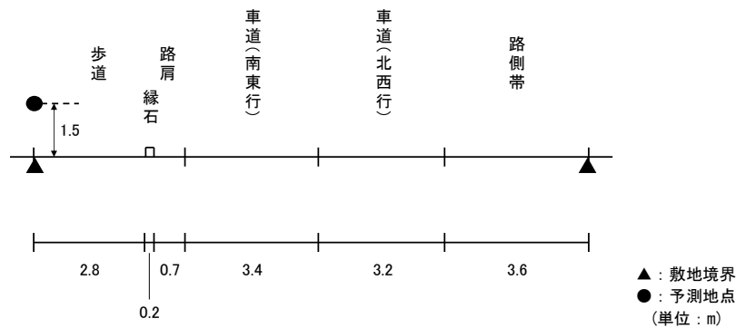
図 11.1-9(2) 予測断面図(予測地点 2 加古川市平岡町高畑・一般国道 2 号)
