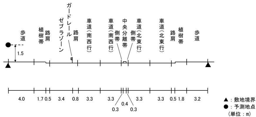
図 11.1-9(8) 予測断面図(予測地点 8 高砂市荒井町東本町・主要地方道 43 号高砂北条線)
