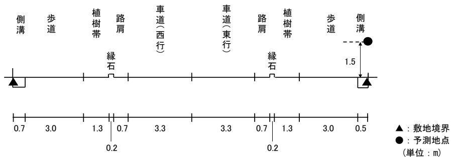
図 11.1-9(20) 予測断面図(予測地点 20 姫路市広畑区長町・一般国道 250 号)
