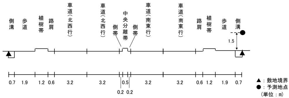
図 11.1-9(13) 予測断面図(予測地点 13 姫路市木場前中町・市道幹第 55 号線)
