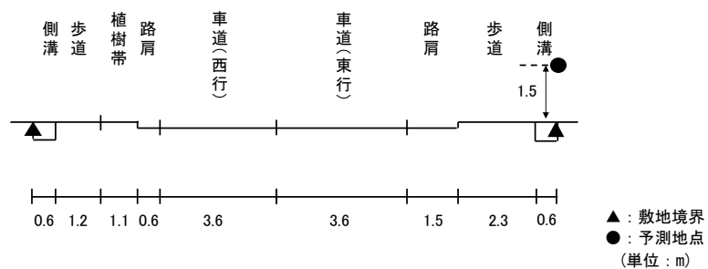
図 11.1-9(19) 予測断面図(予測地点 19 姫路市飾磨区思案橋・一般国道 250 号)
