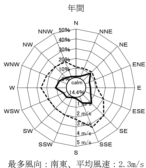
図 11.1-3(2) 気象(風向・風速)の現地調査結果[A-2 加古川市尾上公園]
