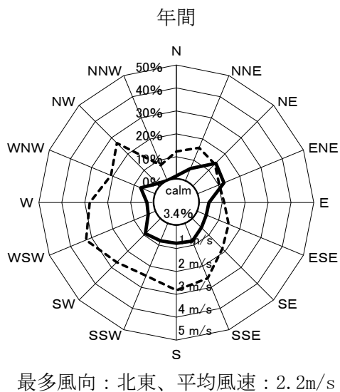
図 11.1-3(1) 気象(風向・風速)の現地調査結果[A-1 加古川市上ノ池公園]
