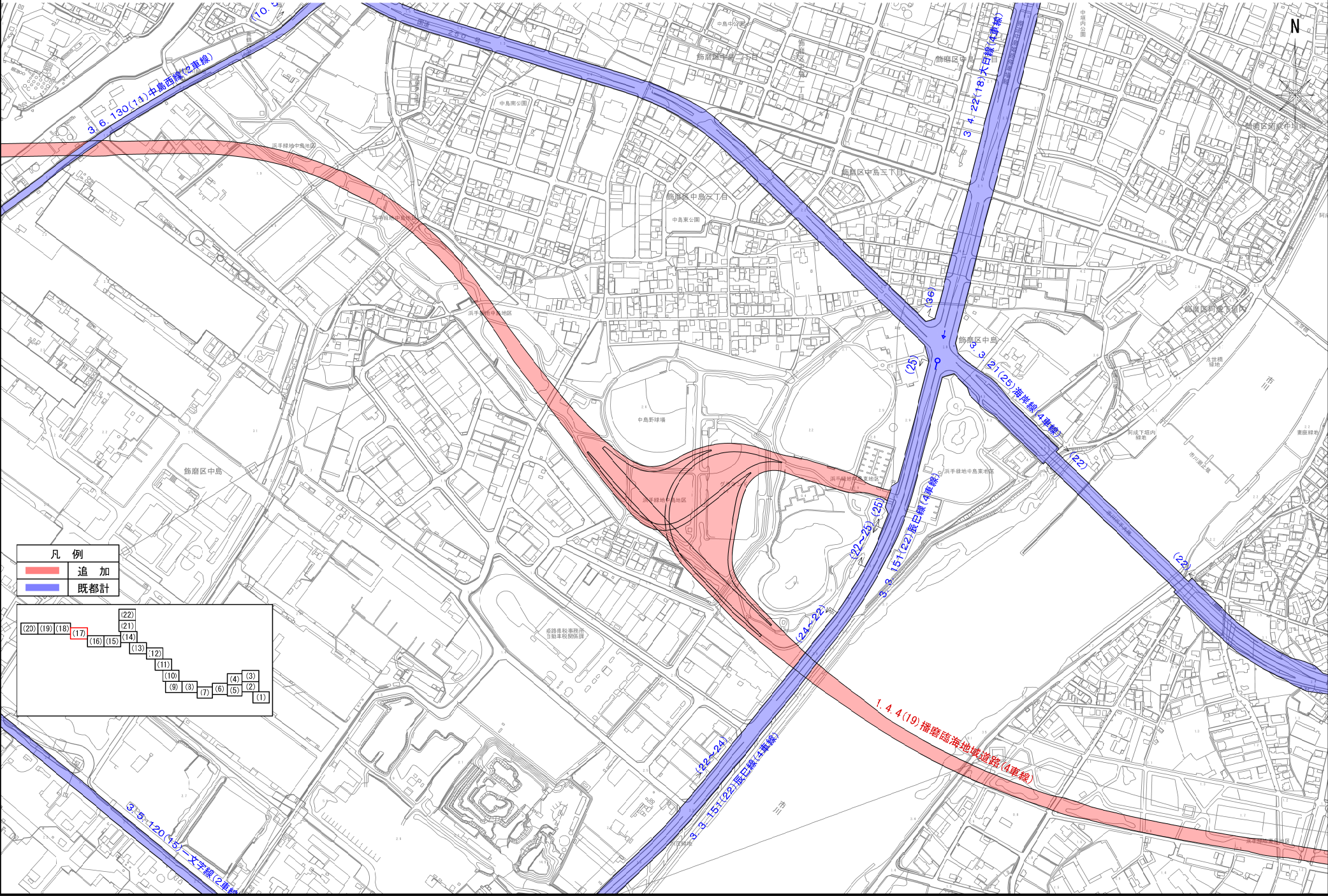
計 画 図(17) S=1:2500
