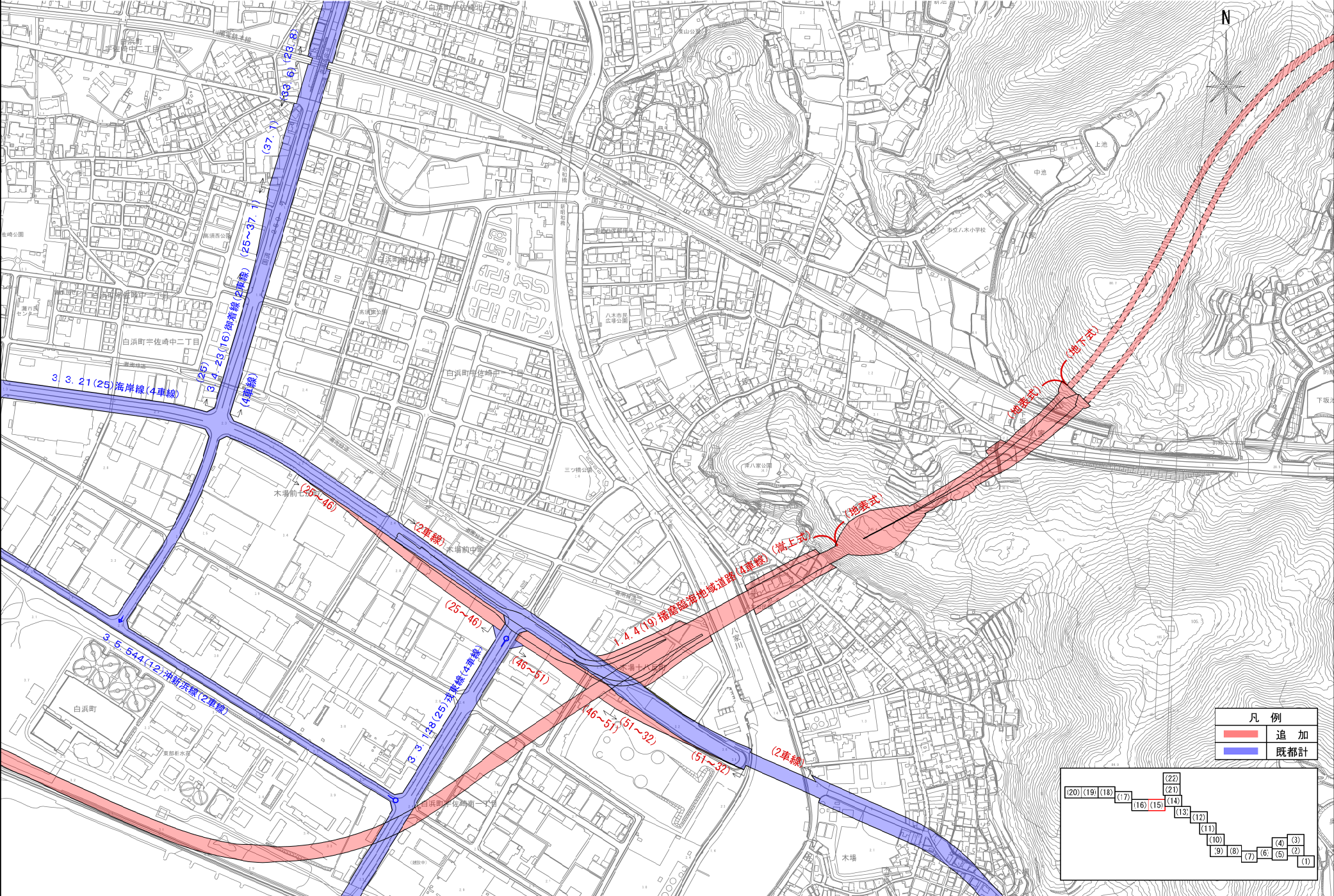
計 画 図(15) S=1:2500
