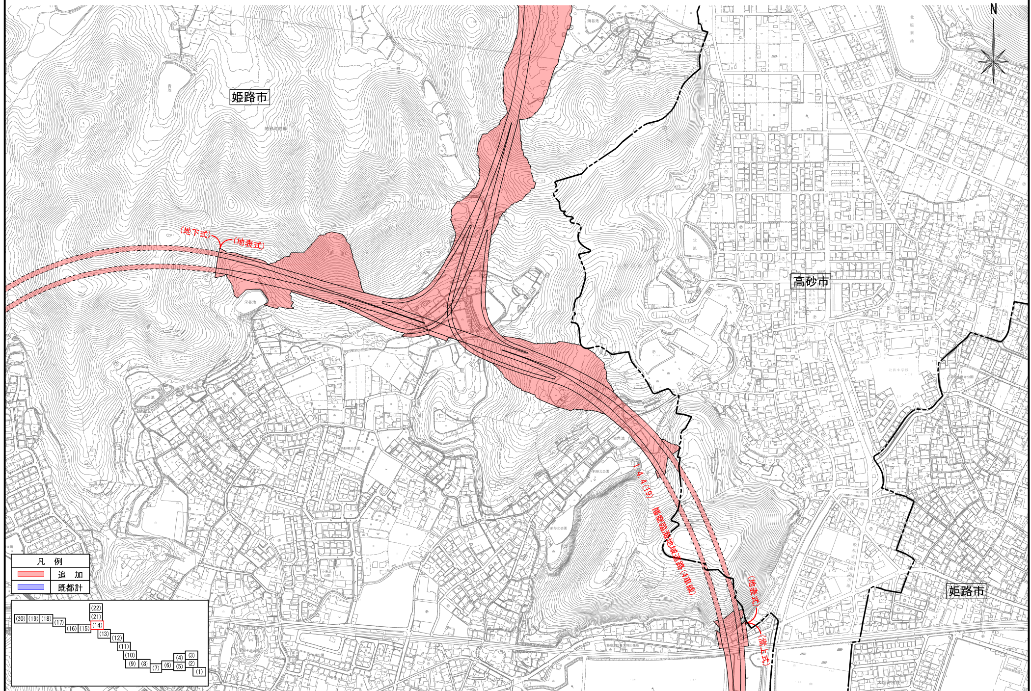
計 画 図(14) S=1:2500
