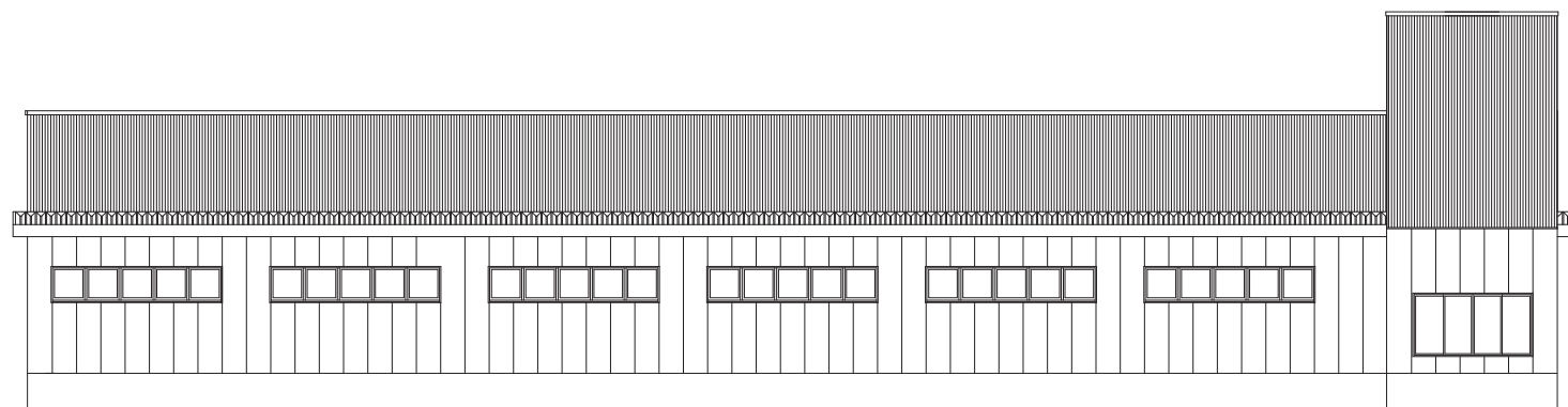
未定物販②棟 東側立面図(1 : 200)
