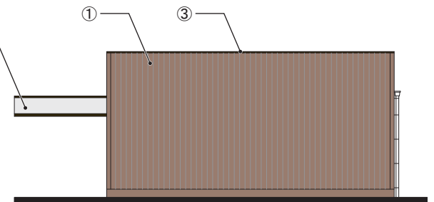
非物販棟 東側立面図(1 : 200)
