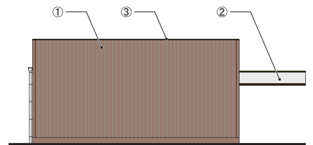
非物販棟 西側立面図(1 : 200)
