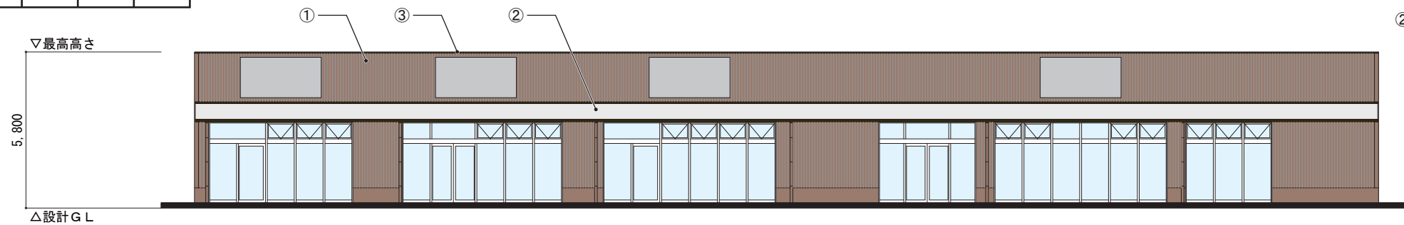
非物販棟 南側立面図(1 : 200)
