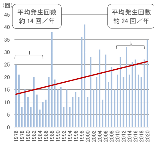
図67 80mm/h以上の降雨年間発生回数の推移(全国)
