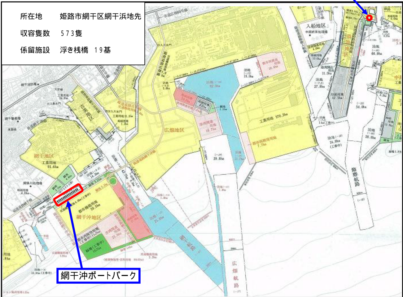
姫路港網干ポートパーク 平面図
