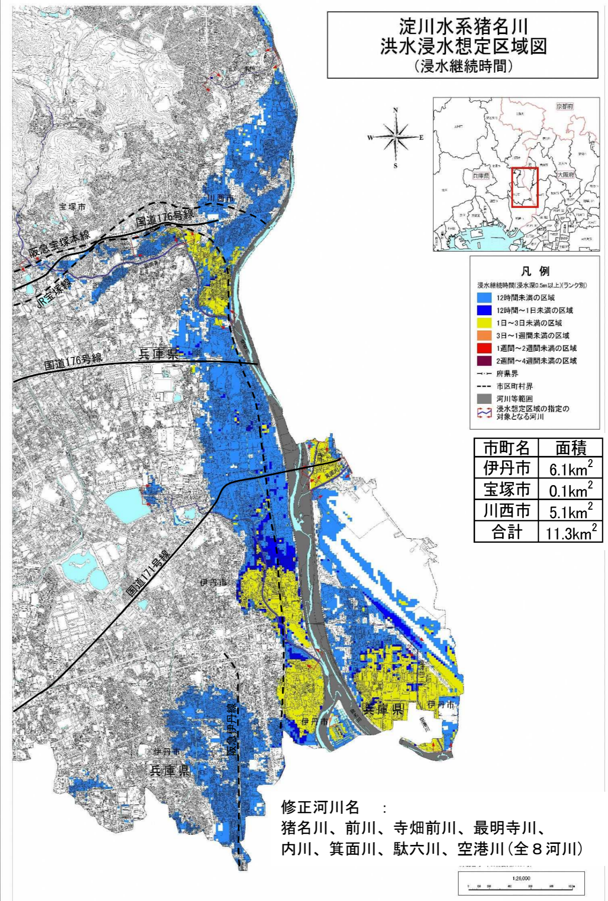
【修正後】浸水継続時間図
