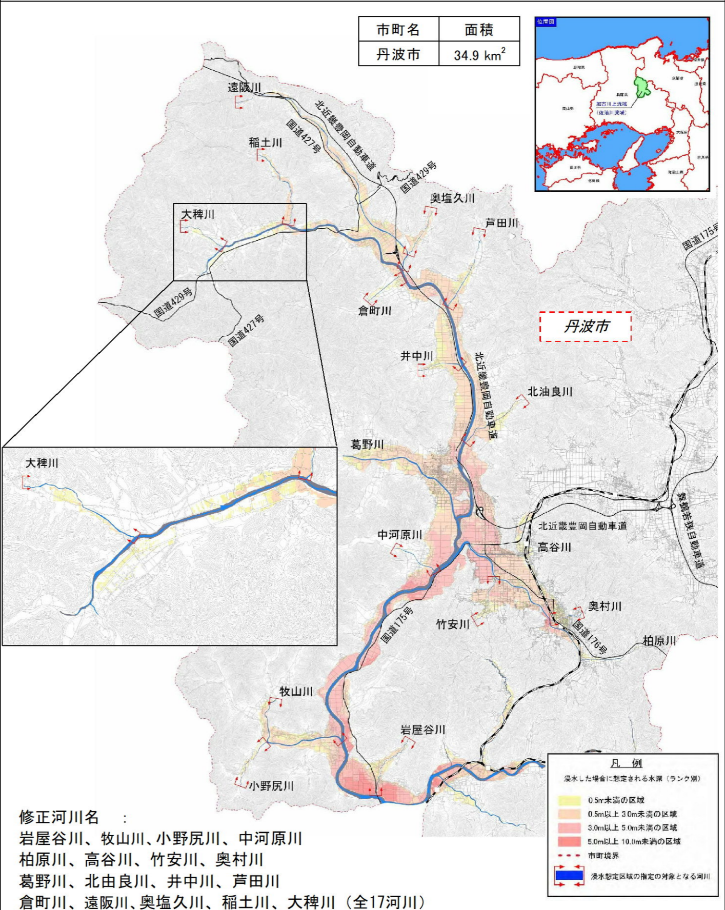
【修正後】洪水浸水想定区域図(浸水深【想定最大規模】)
