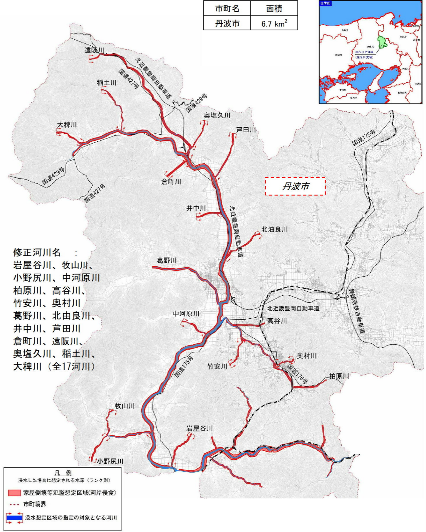
【修正後】洪水浸水想定区域図(河岸侵食)
