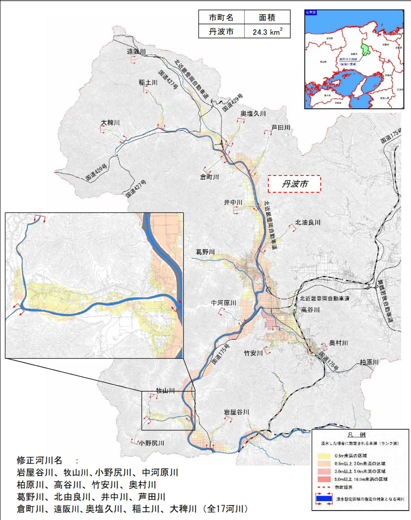
【修正後】洪水浸水想定区域図(浸水深【計画規模】)
