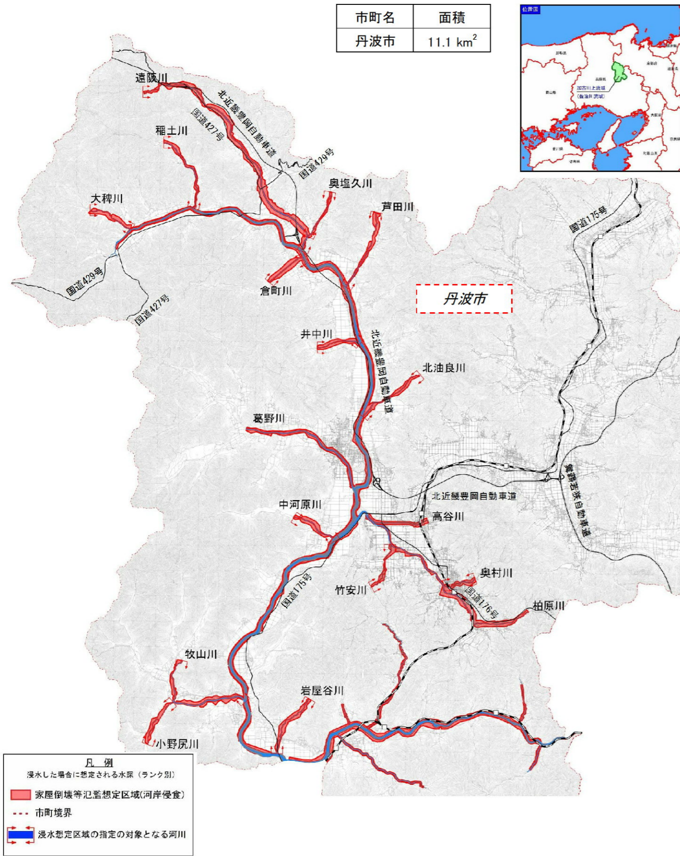
【修正前】洪水浸水想定区域図(河岸侵食)
