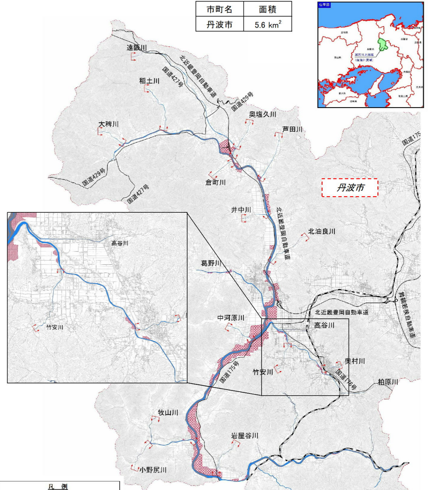
【修正後】洪水浸水想定区域図(氾濫流)
