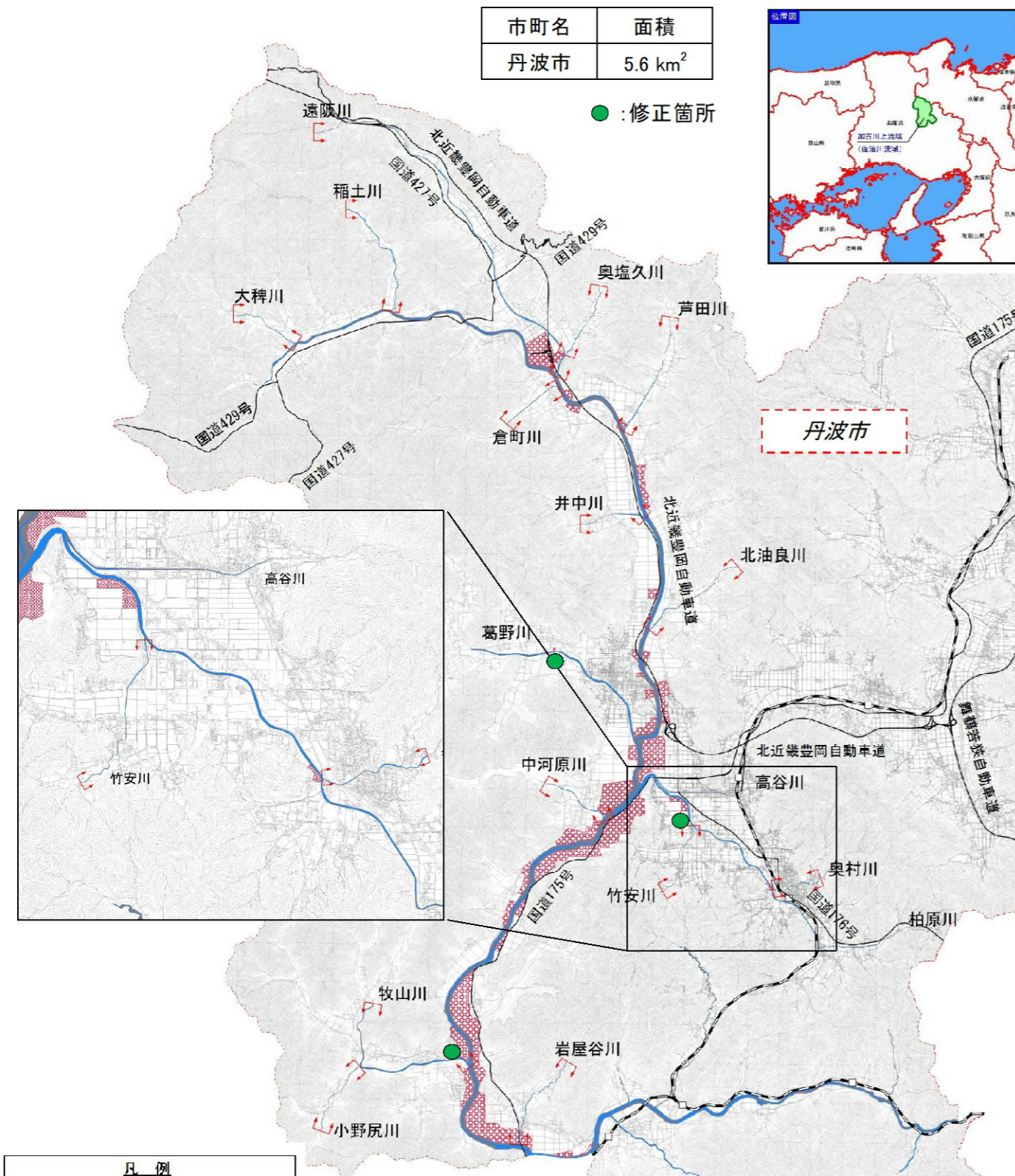
【修正前】洪水浸水想定区域図(氾濫流)
