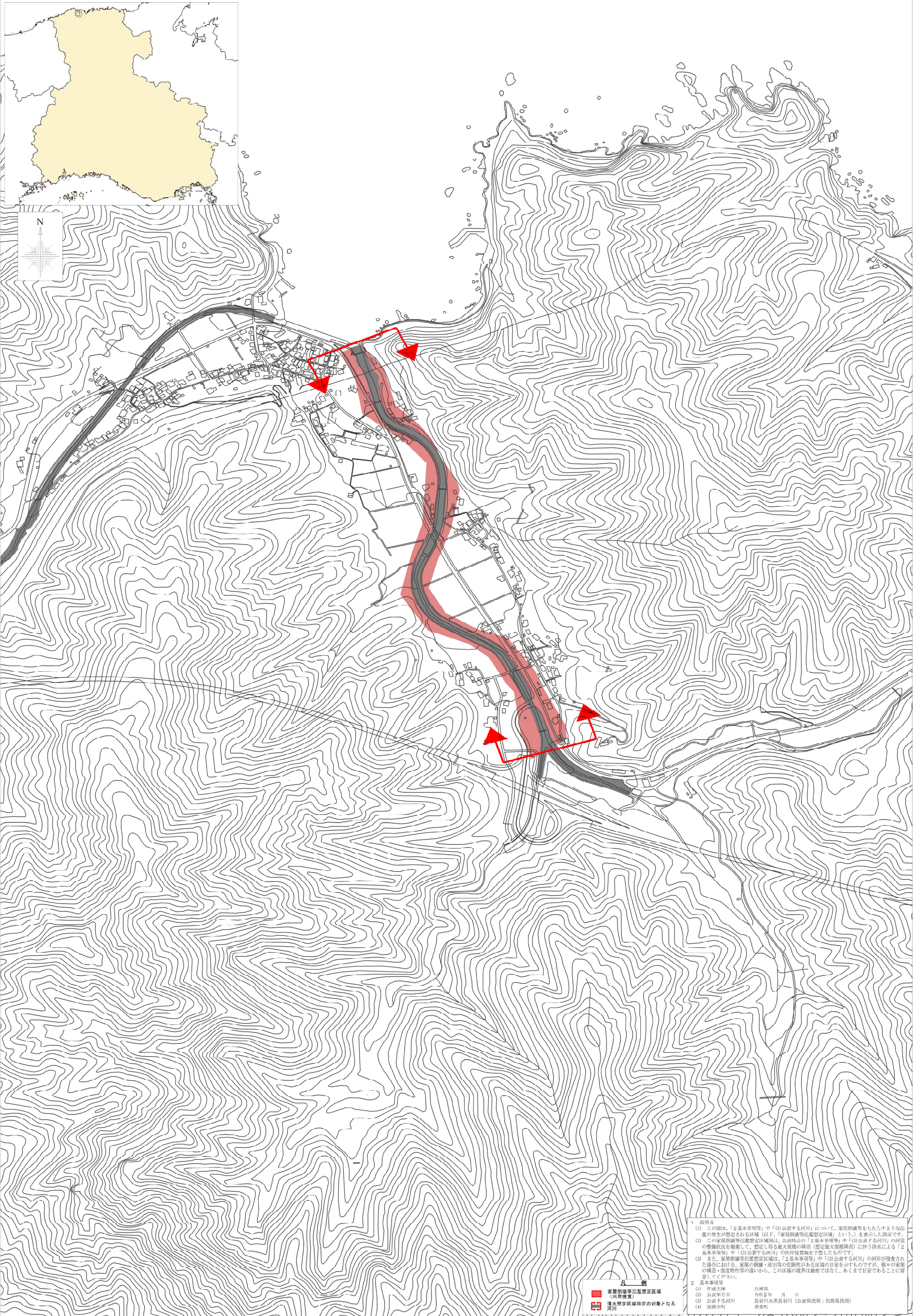
長谷川水系長谷川 家屋倒壊等氾濫想定区域図 河岸侵食
