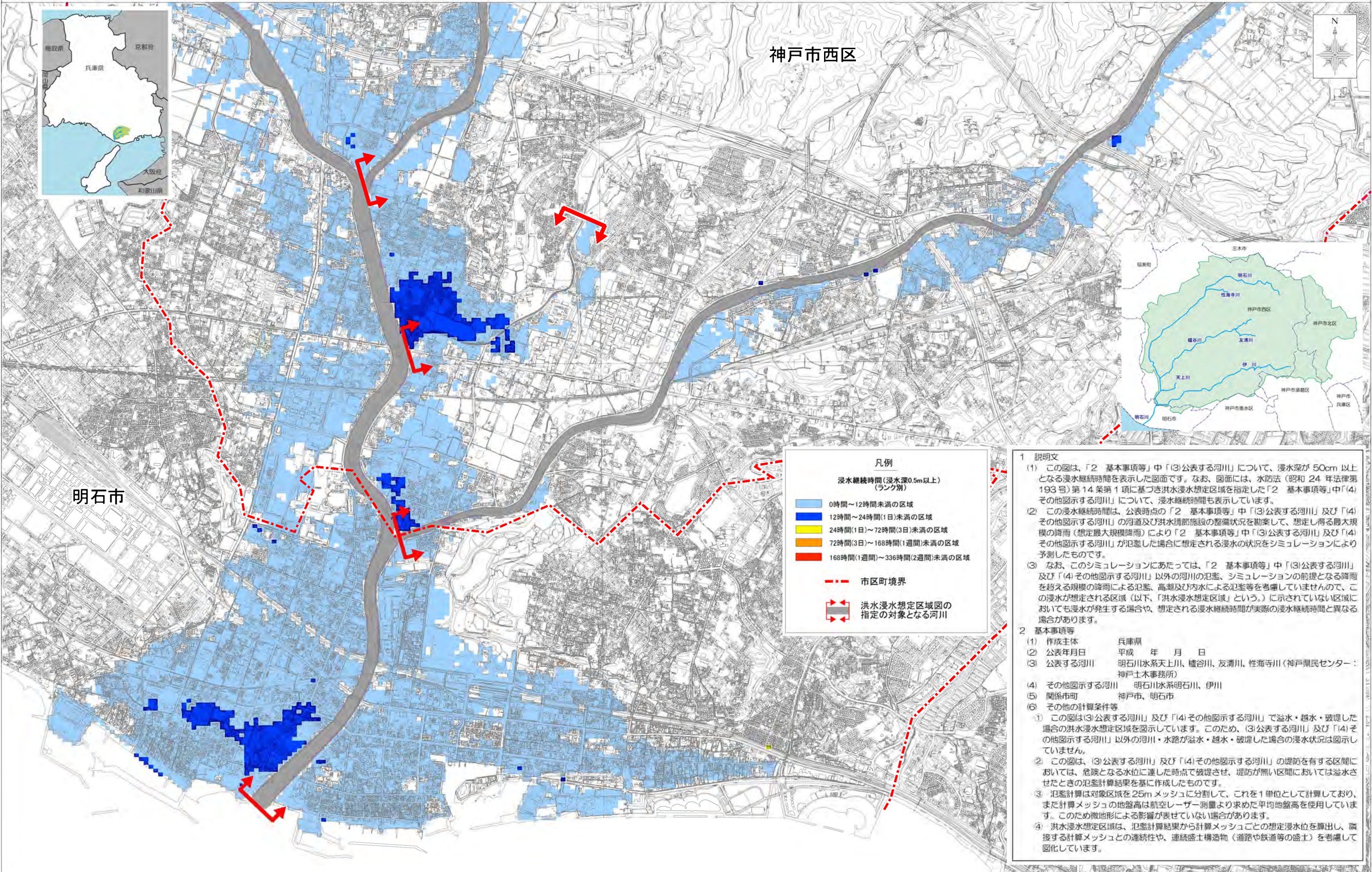
明石川水系 洪水浸水想定区域図(浸水継続時間 1/5)
