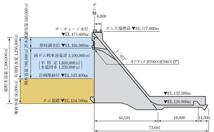
北富士ダム標準断面図
