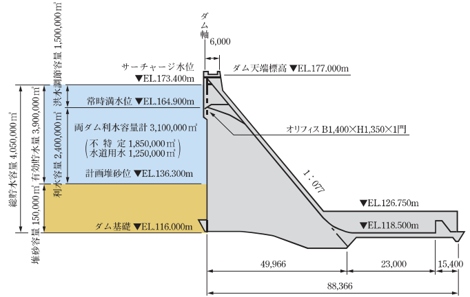
成相ダム標準断面図
