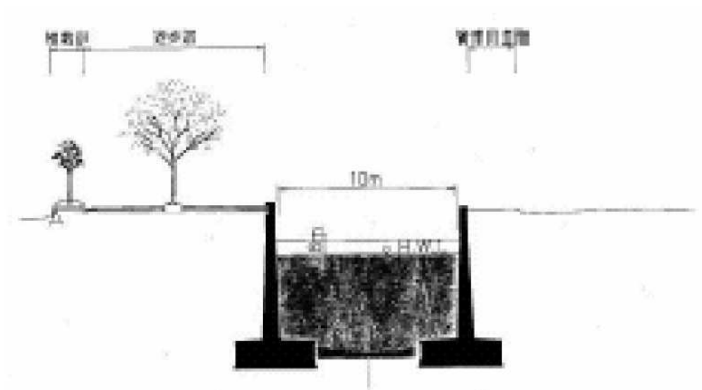
図-2.1.2 流下能力向上対策 イメージ図 (石井川と天王谷川合流点より荻藻川合流点：延長 2,503m)
