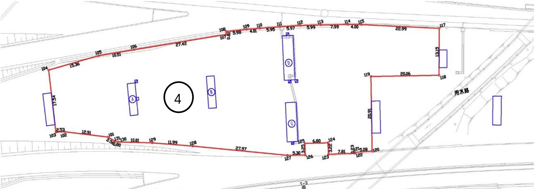
(2) 平面図・求積表 (物件番号: ④)
