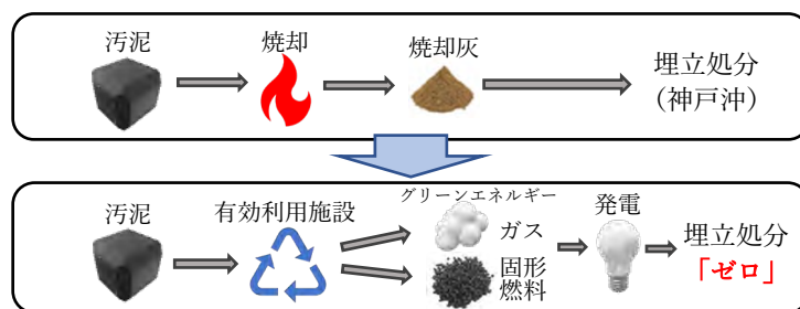
下水汚泥からグリーンエネルギー生成イメージ図
