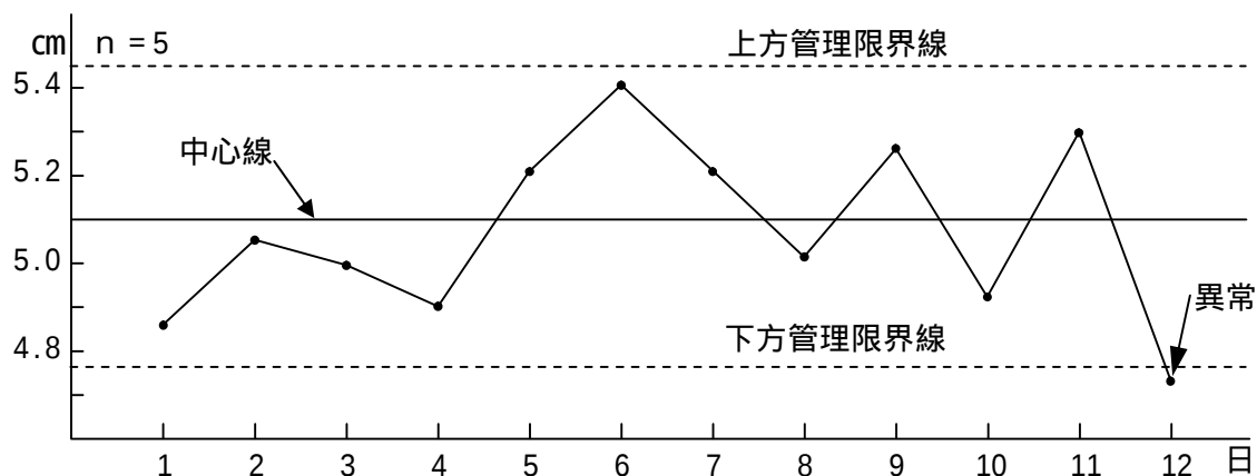
図 - 10 管 理 図
