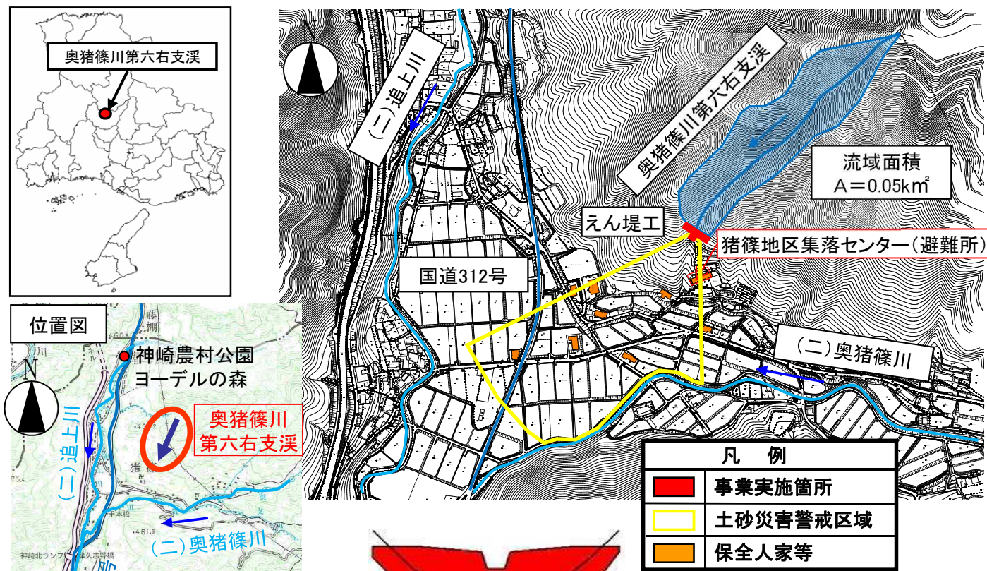
えん堤工 H=7.0m L=40.0m
