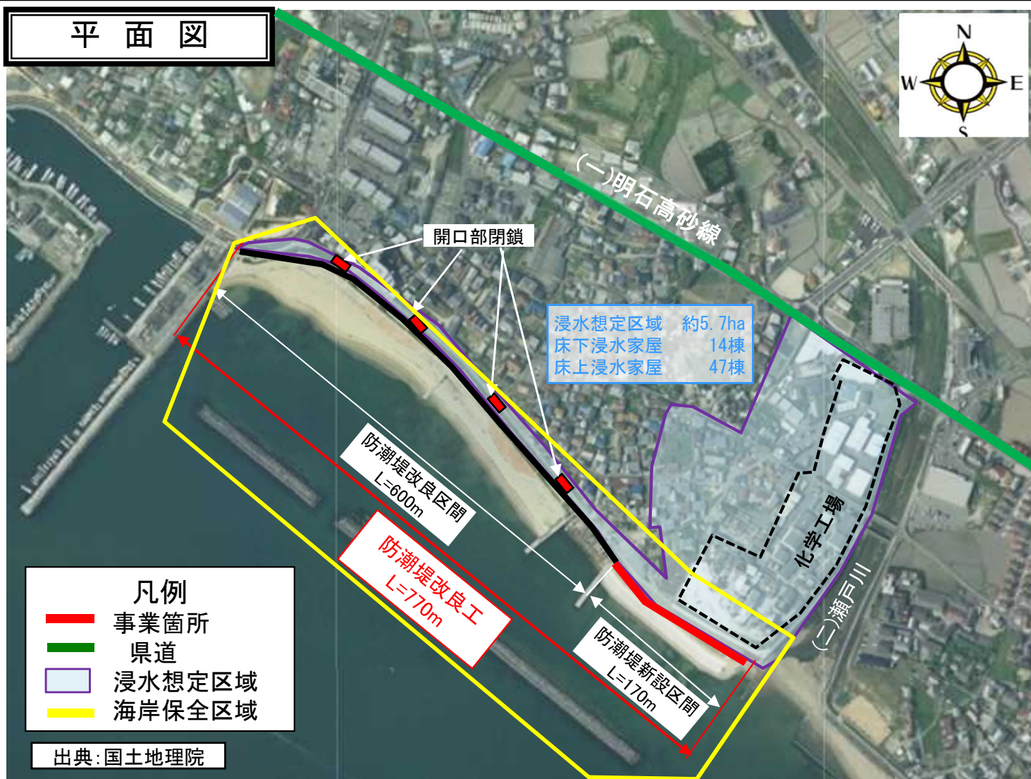
防潮堤新設区間
