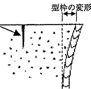
—型枠の変形—
