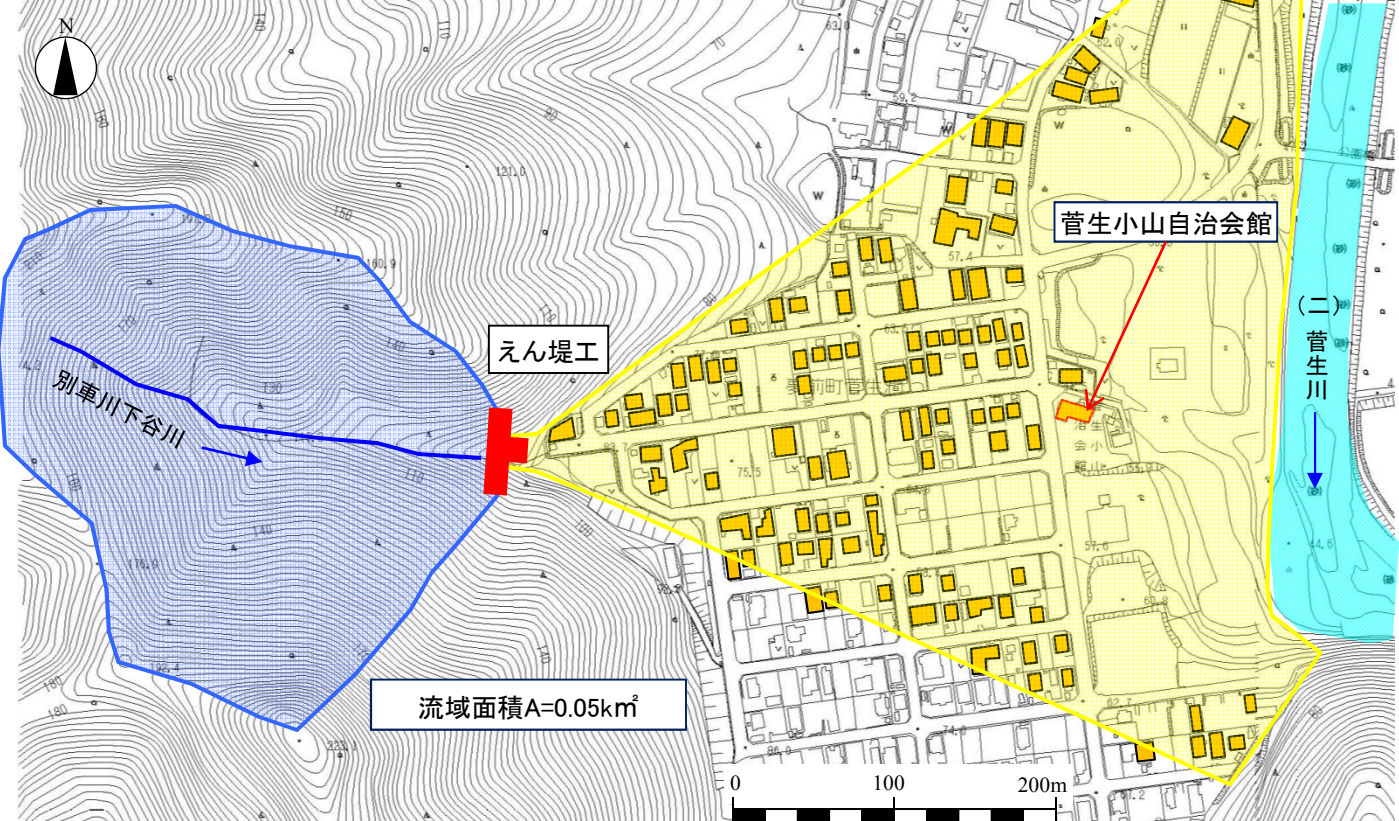
えん堤工 H=7.0m、L=65.0m
