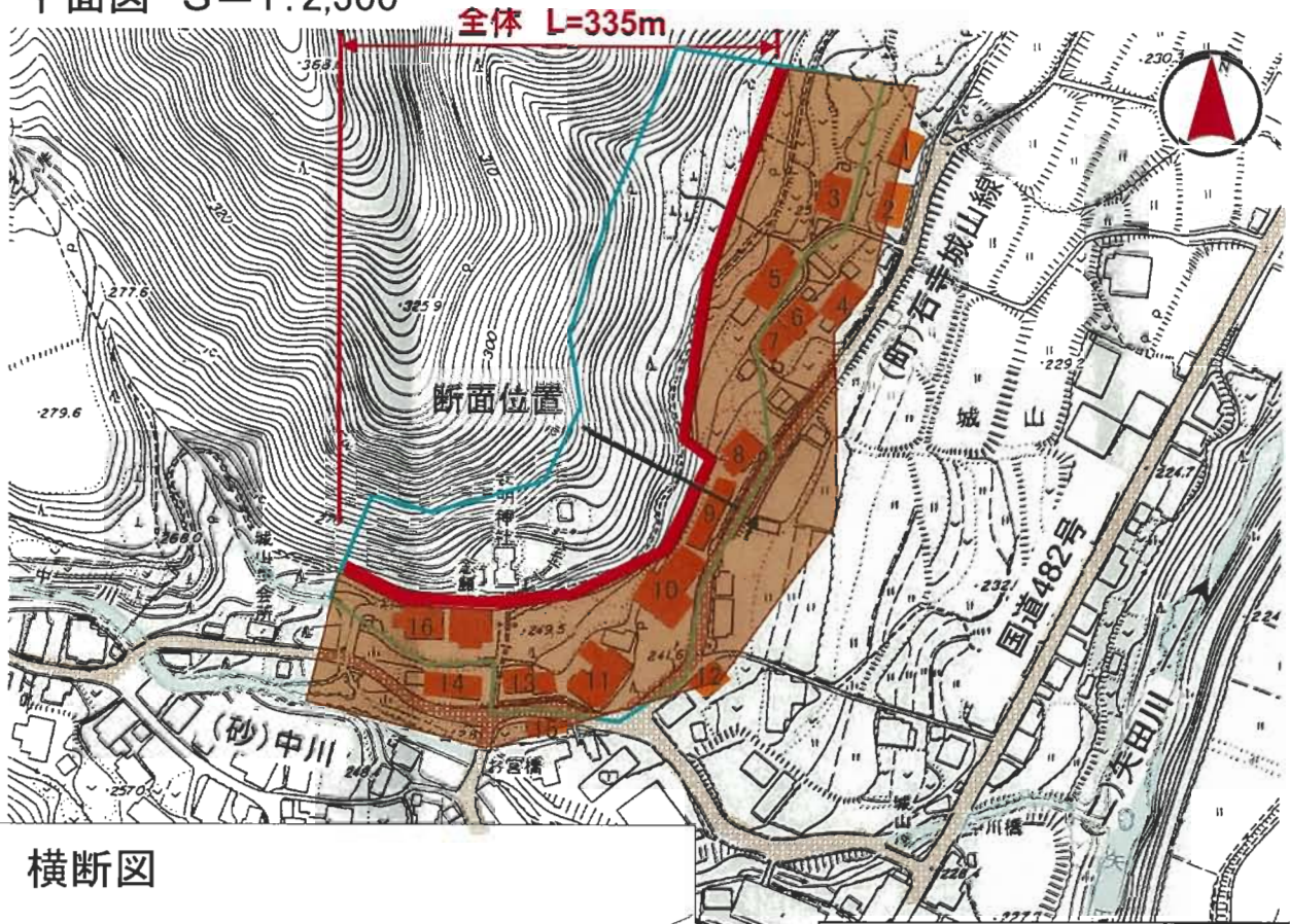
平面図 S=1:2,500
