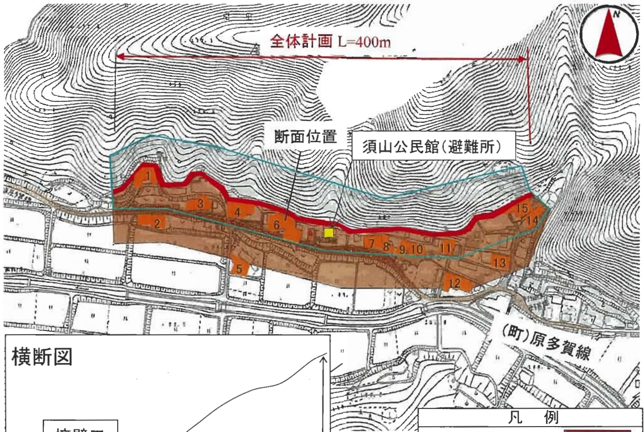
平面図 S=1:2,500
