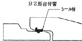
BZ 形台付管：管の受け口に予めシール材が埋込まれた構造（ガスケットタイプ）
