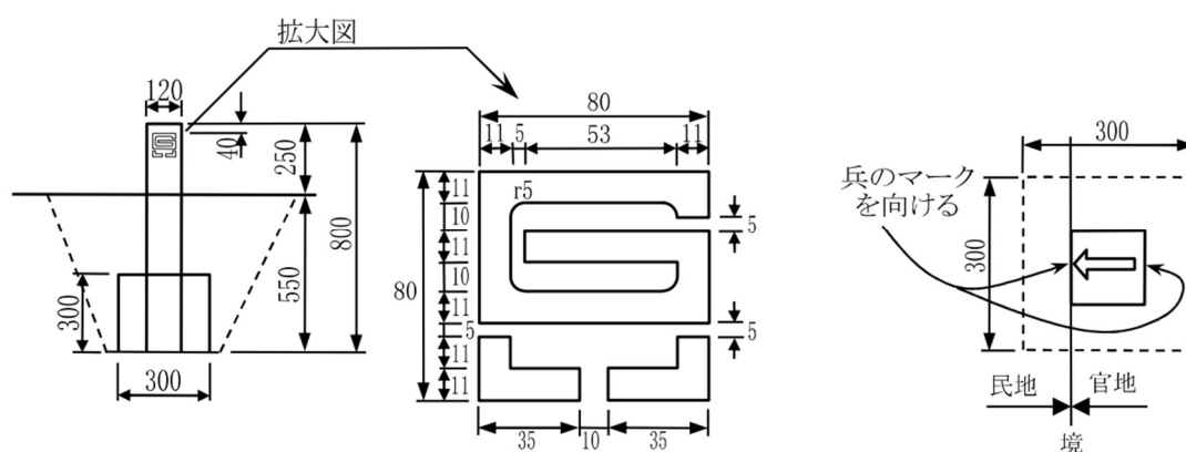
図 6-1-1 境界杭(鈎)の設置
