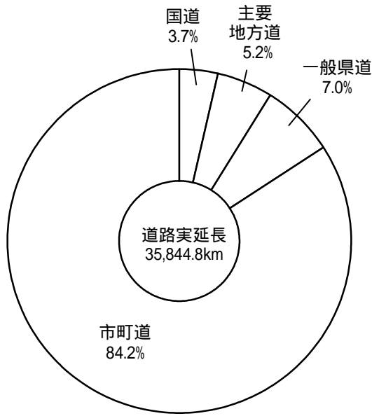
道路実延長の道路種別割合 (平成23年4月1日現在)
