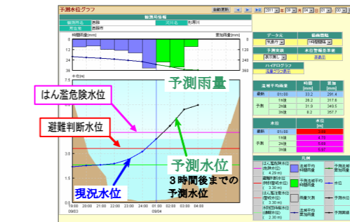
図7-6 水位予測（フェニックス防災システム）
