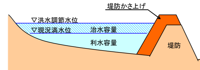
堤防の嵩上げによる治水容量の確保
