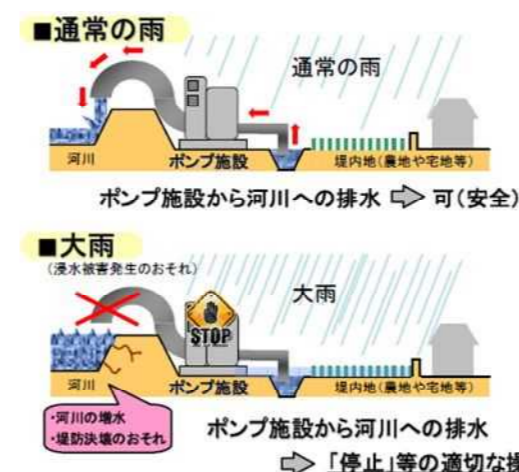
図 6-7 排水ポンプの運転調整
