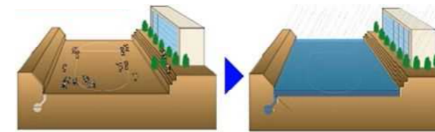
図 6-1 校庭貯留
