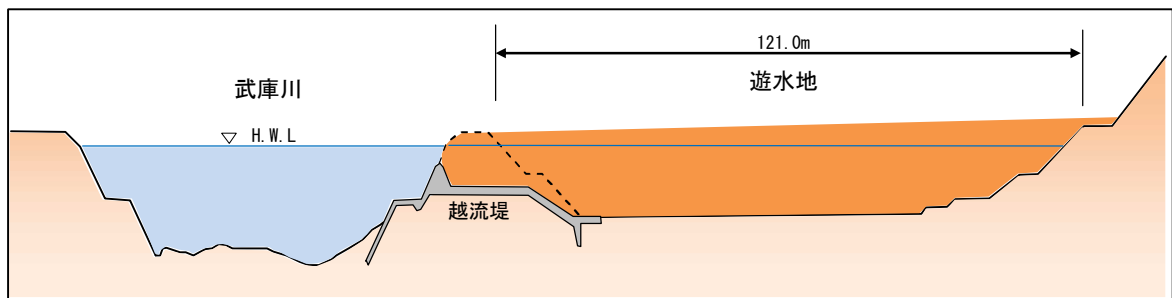
図 5-6 武庫川遊水地の構造図
