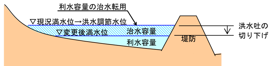
図 6-4 ため池貯留
