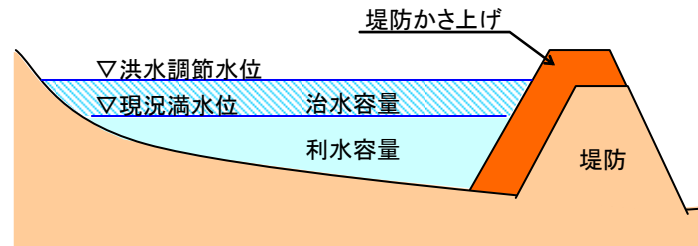
図 6-4 ため池貯留
