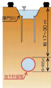
図 5-4 地下貯留管のイメージ図
