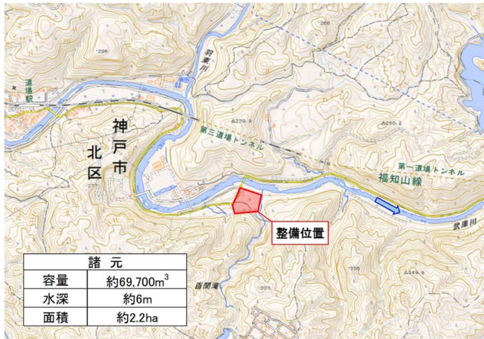
図 5-5 整備の場所
