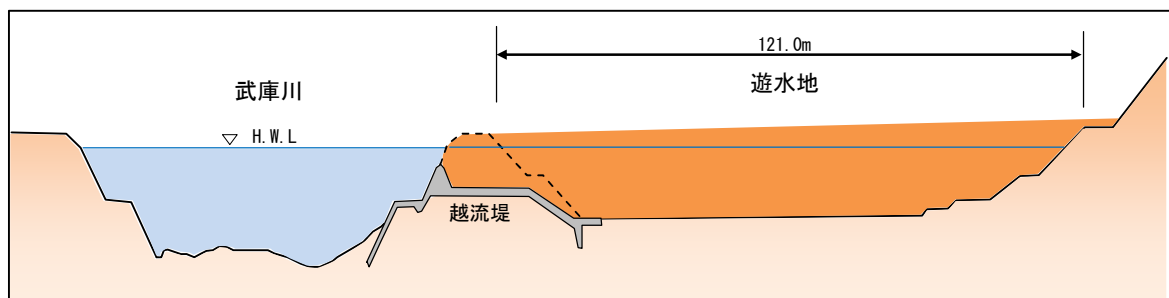
図 5-6 新規遊水地武庫川遊水地の構造図
