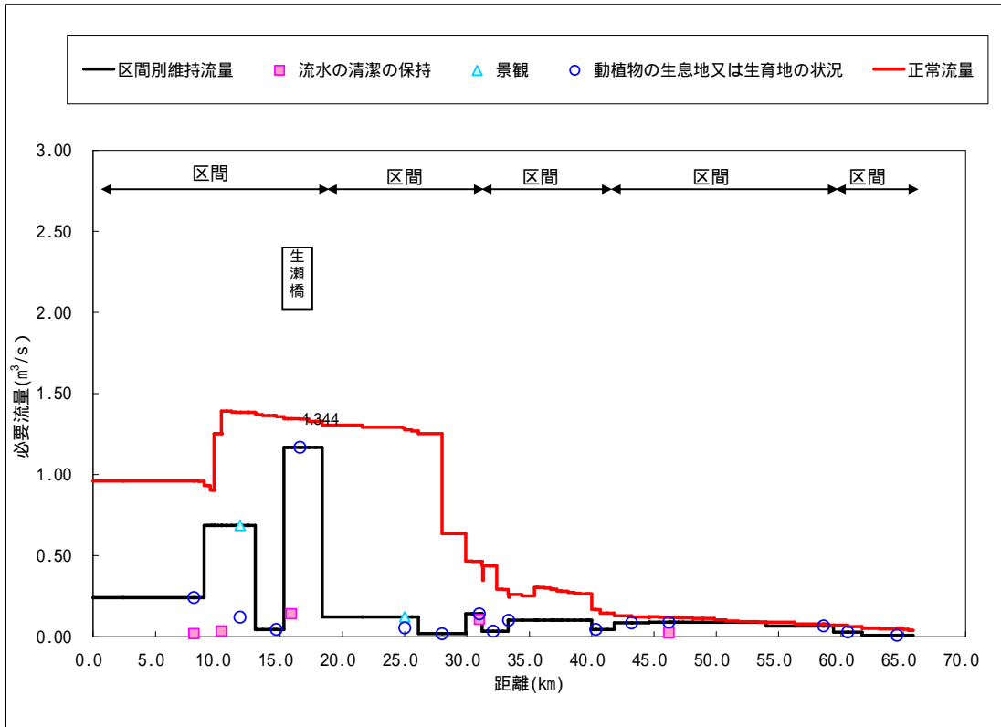
図 5.2(9) 武庫川正常流量(期間：12/1～12/31)
