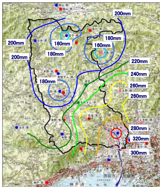
図 4.2.1 昭和58年9月27日洪水の等雨量線図
