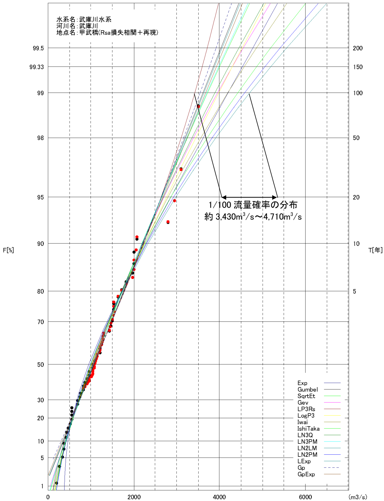
図 2.5 流量確率分布図 (将来土地利用)
