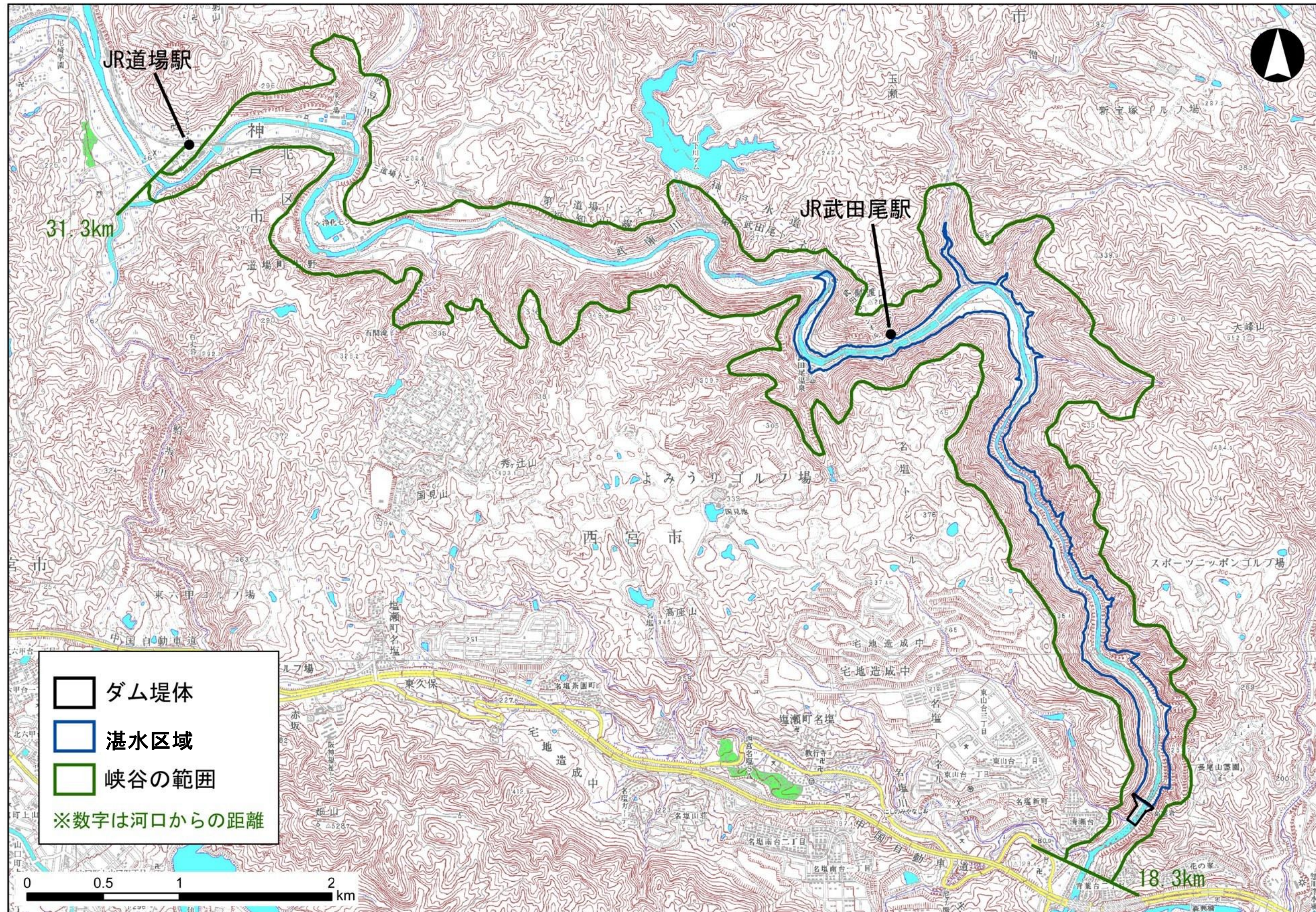
武庫川峡谷 平面図
