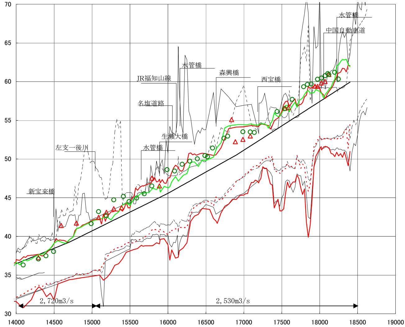
平成16年台風23号痕跡水位縦断面図 (3/3)
