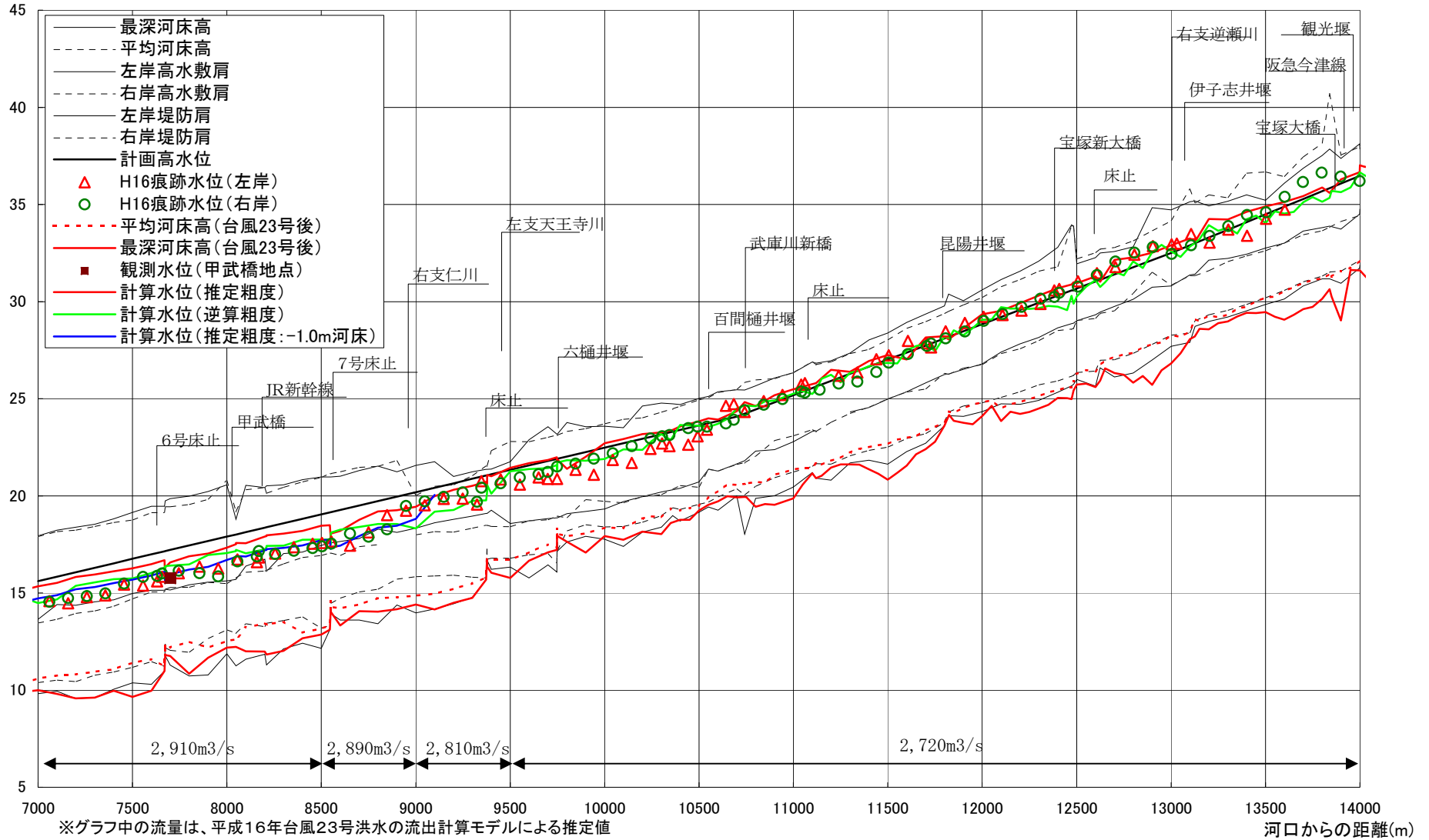
平成16年台風23号痕跡水位縦断図 (2/3)
